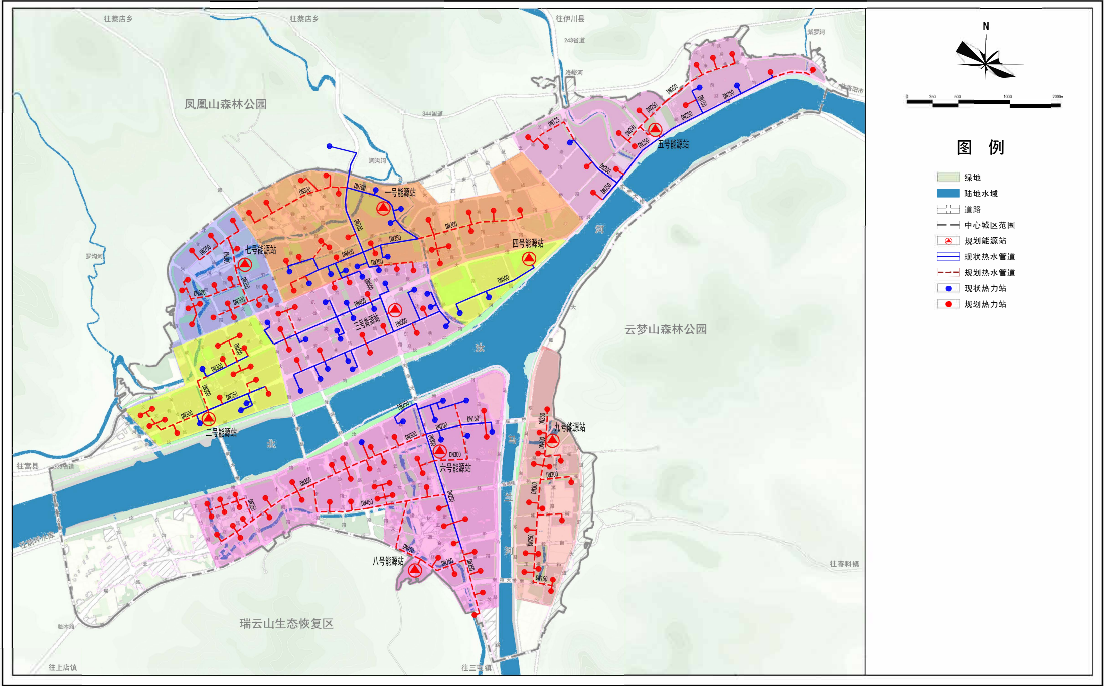
供热工程规划图
