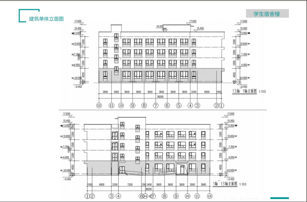
宿舍楼立面图
