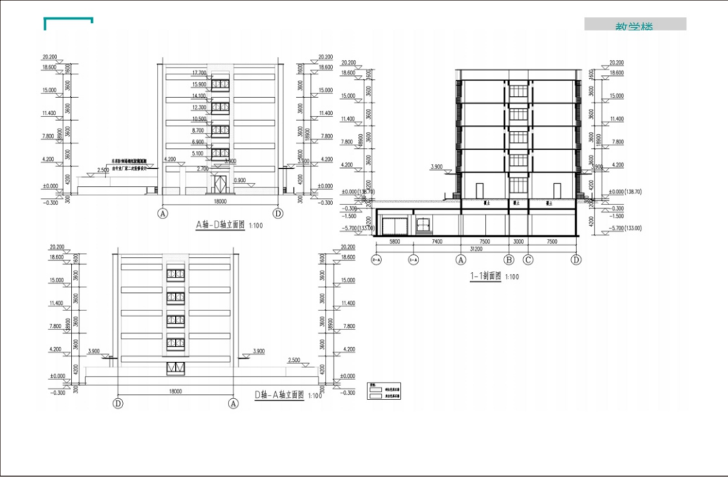
教学楼剖面图
