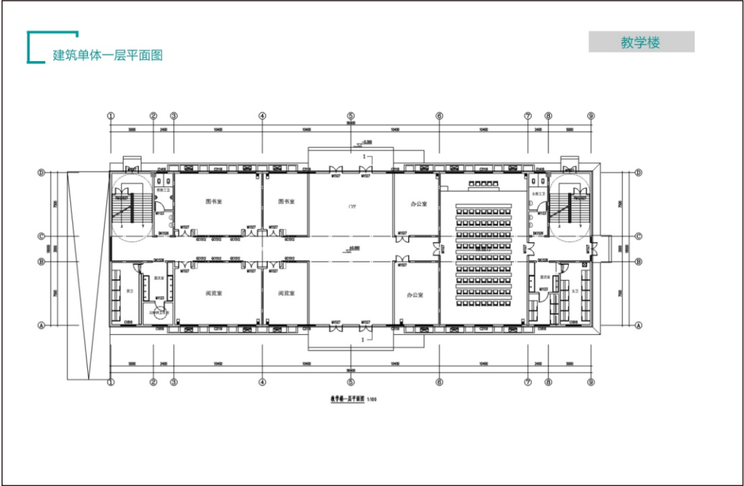
教学楼一层平面图
