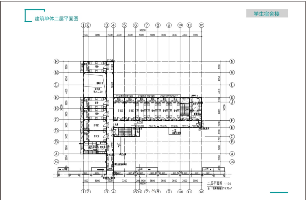
宿舍楼二层平面图
