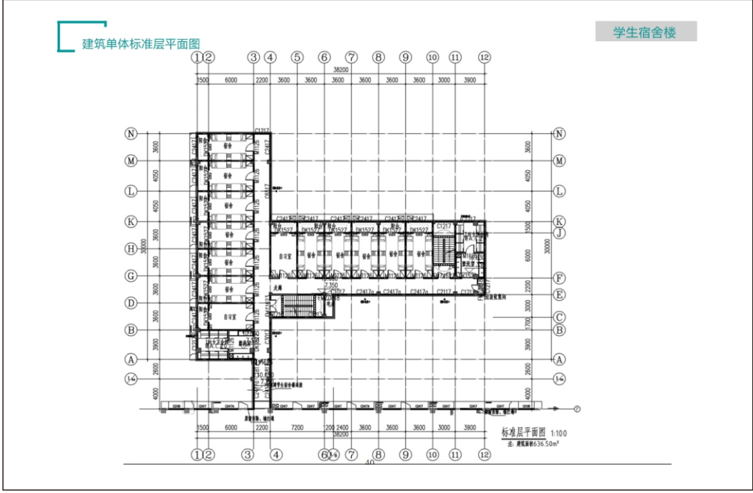
宿舍楼标准平面图
