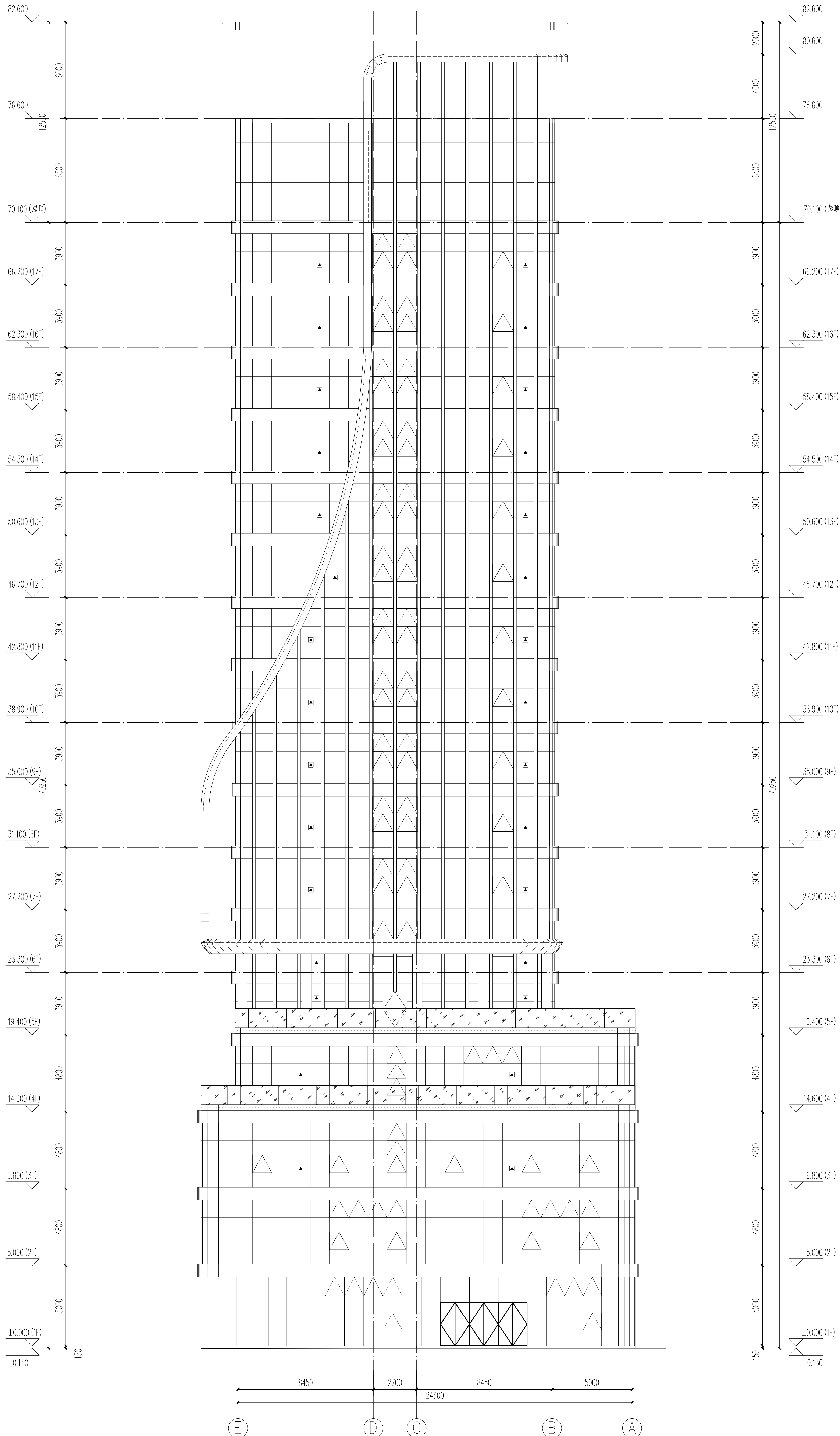
E~A立面图
