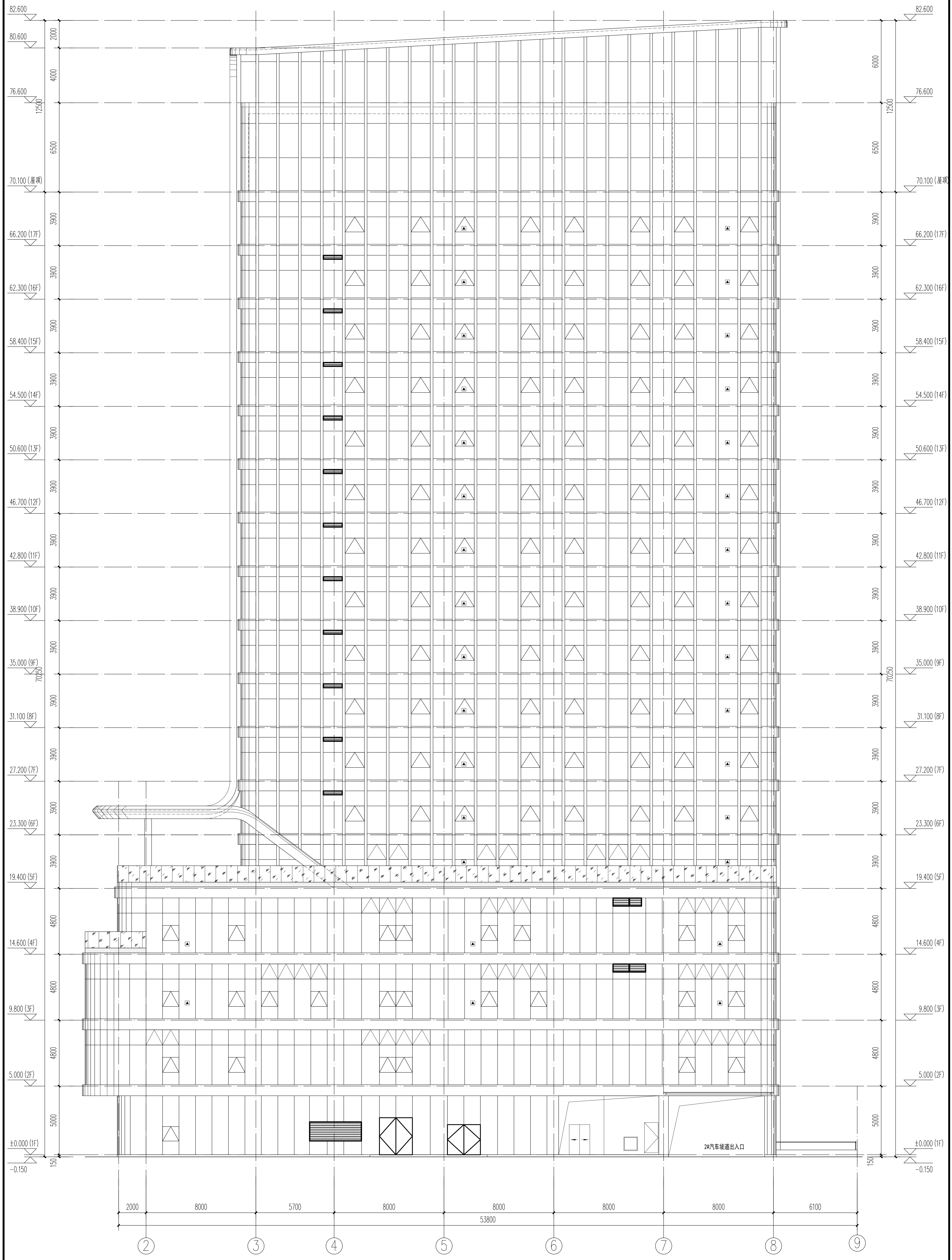
②~⑨立面图
