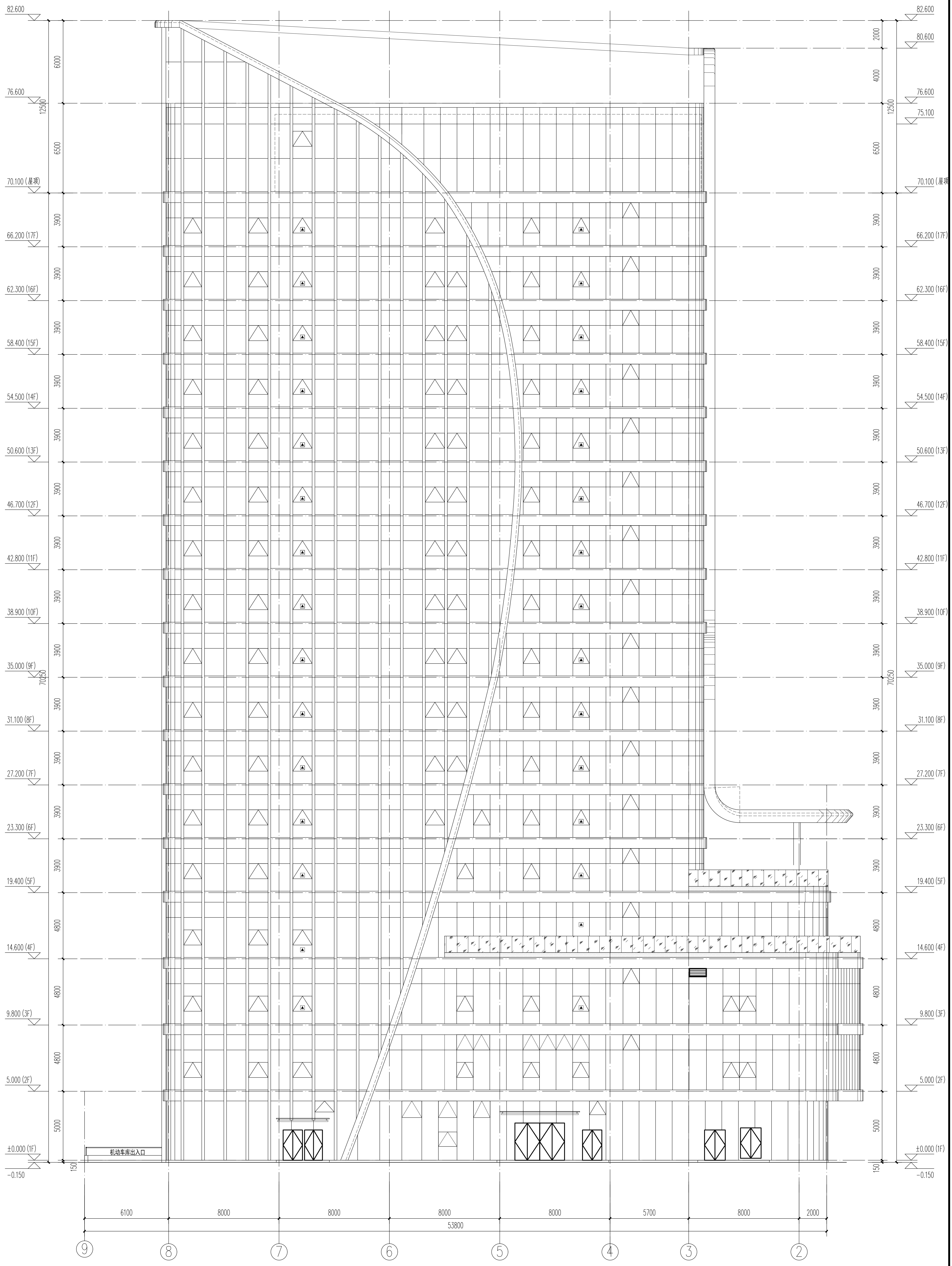
8~2立面图
