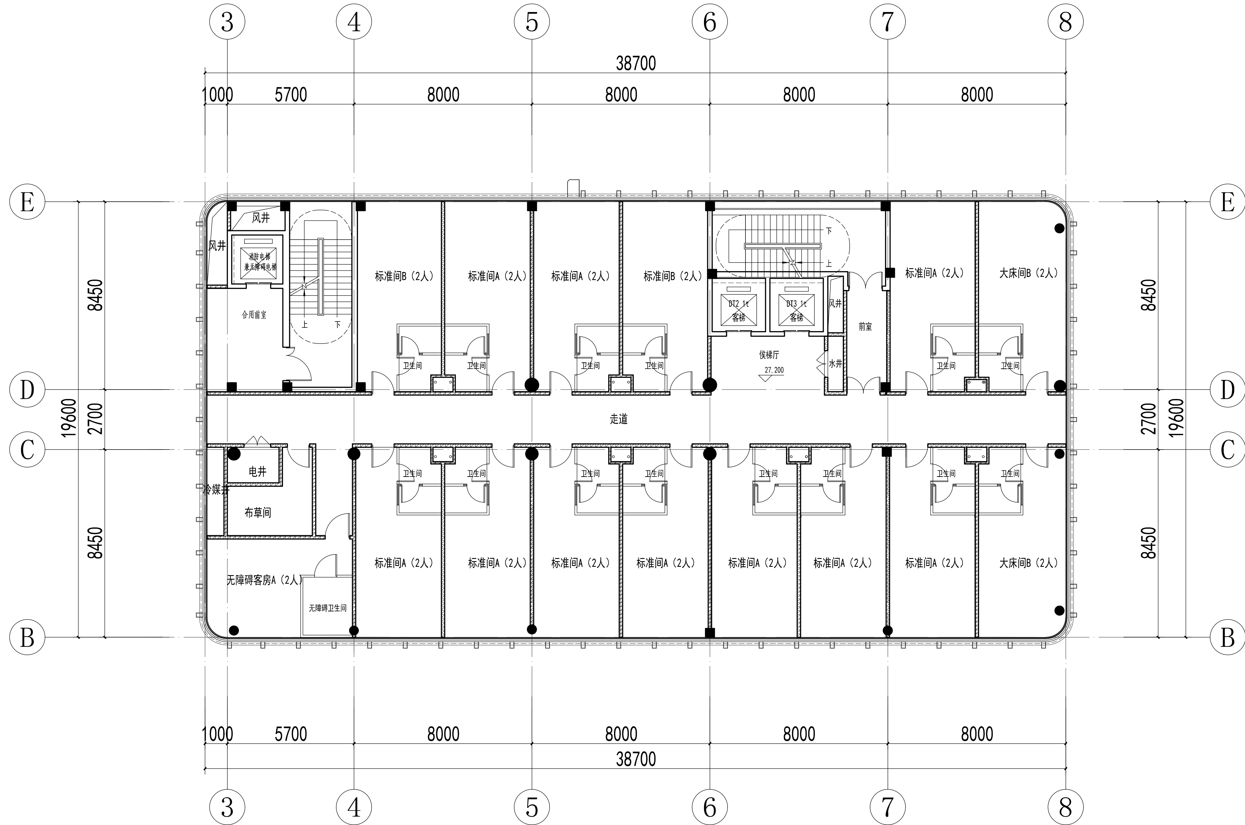
七层平面图
