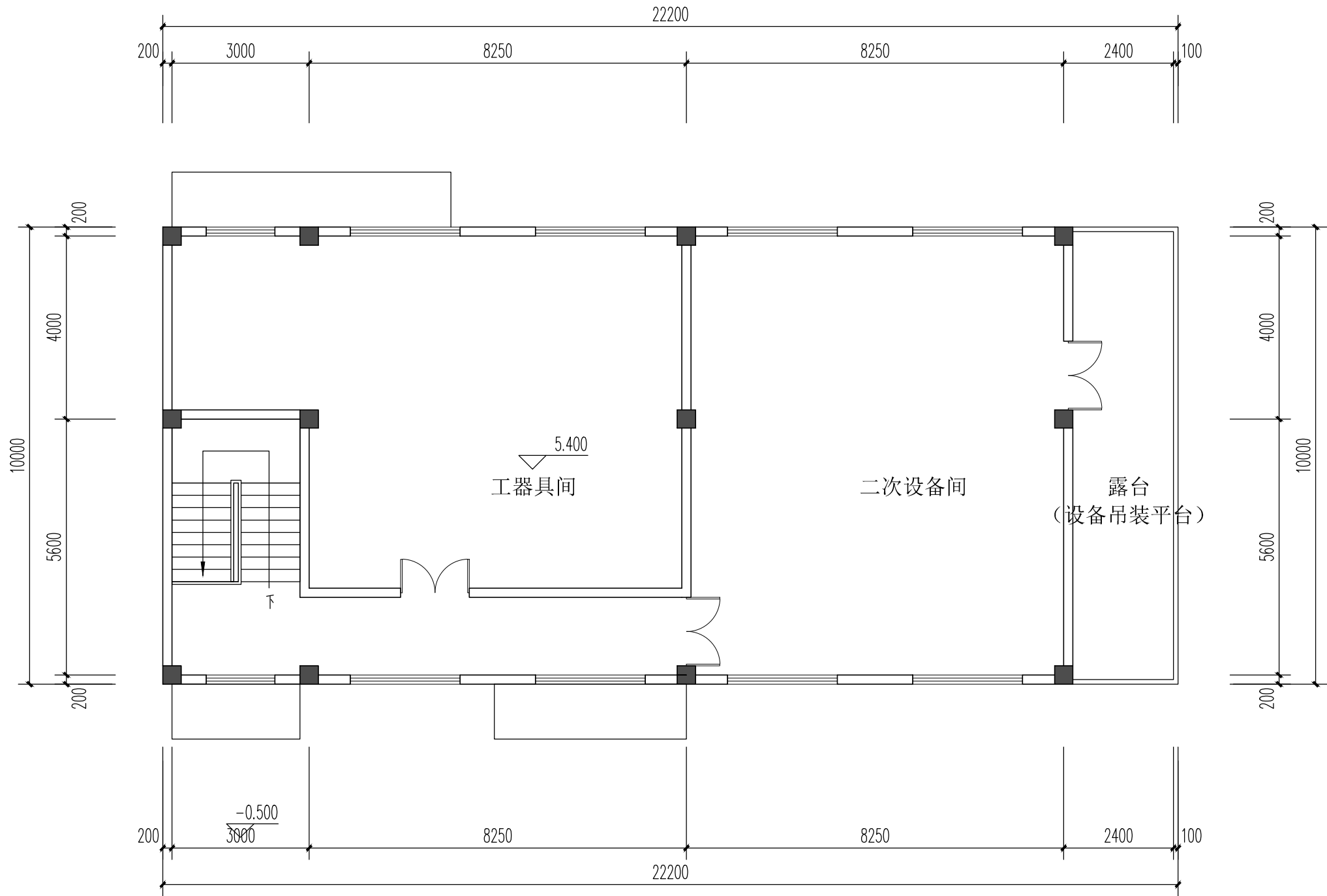
二层平面图 1:100 本层建筑面积: 199.00m 2
