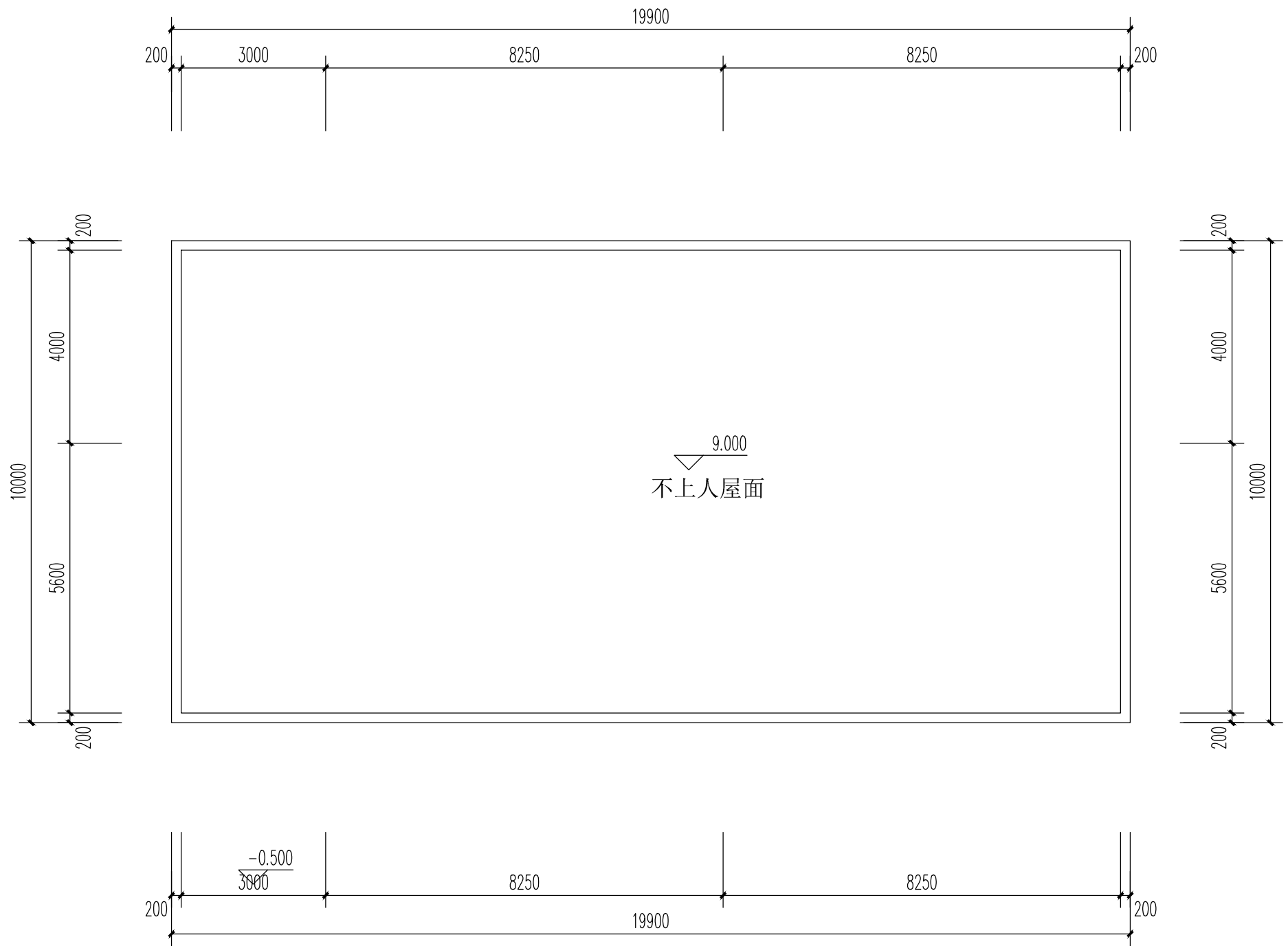
屋顶平面图 1:100
