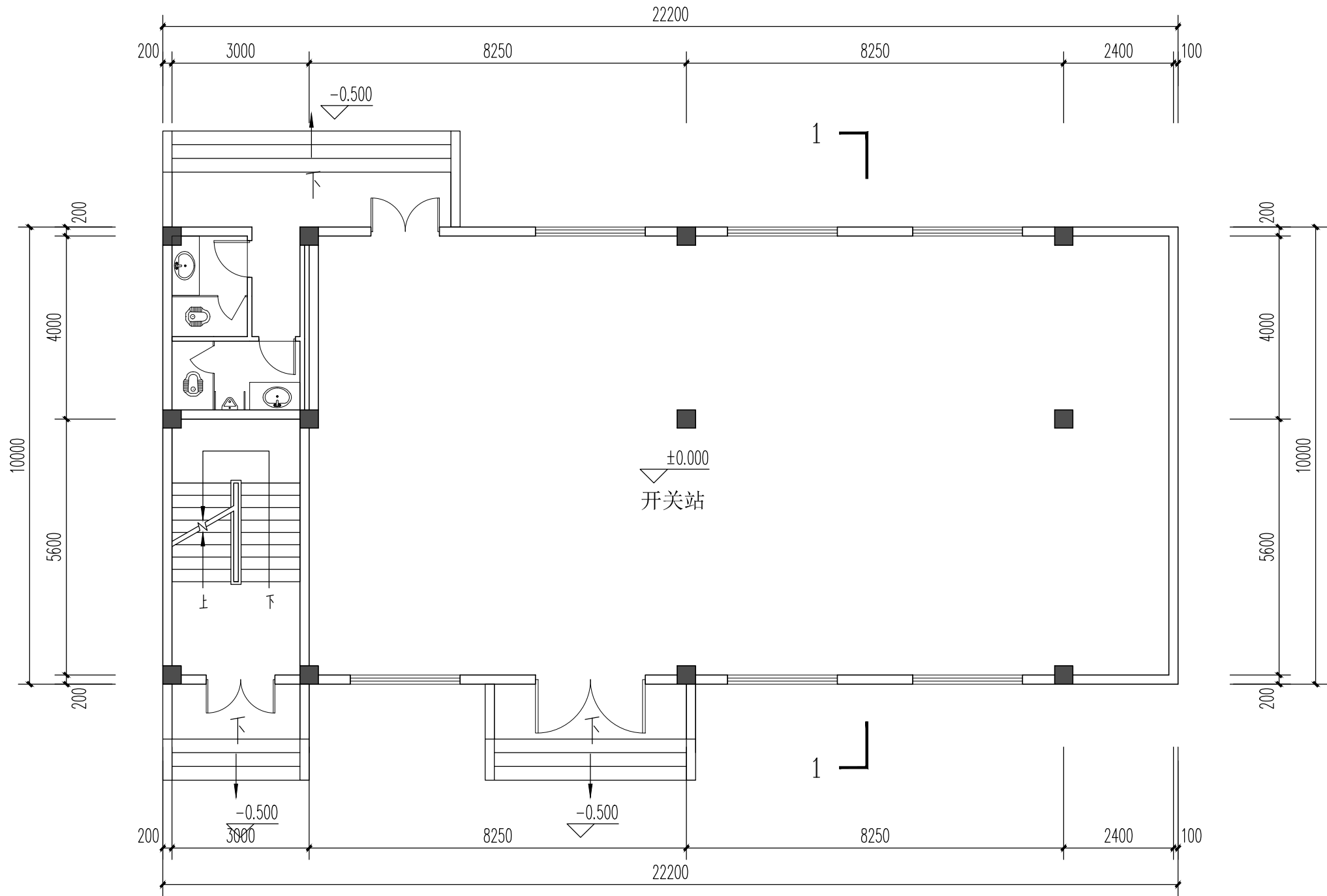
一层平面图 1:100 本层建筑面积: 222.00m 2
