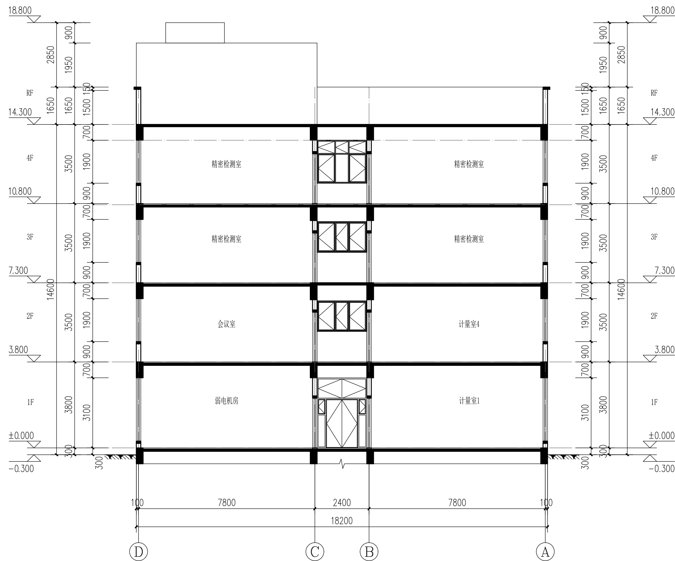
1-1剖面图 1:100
