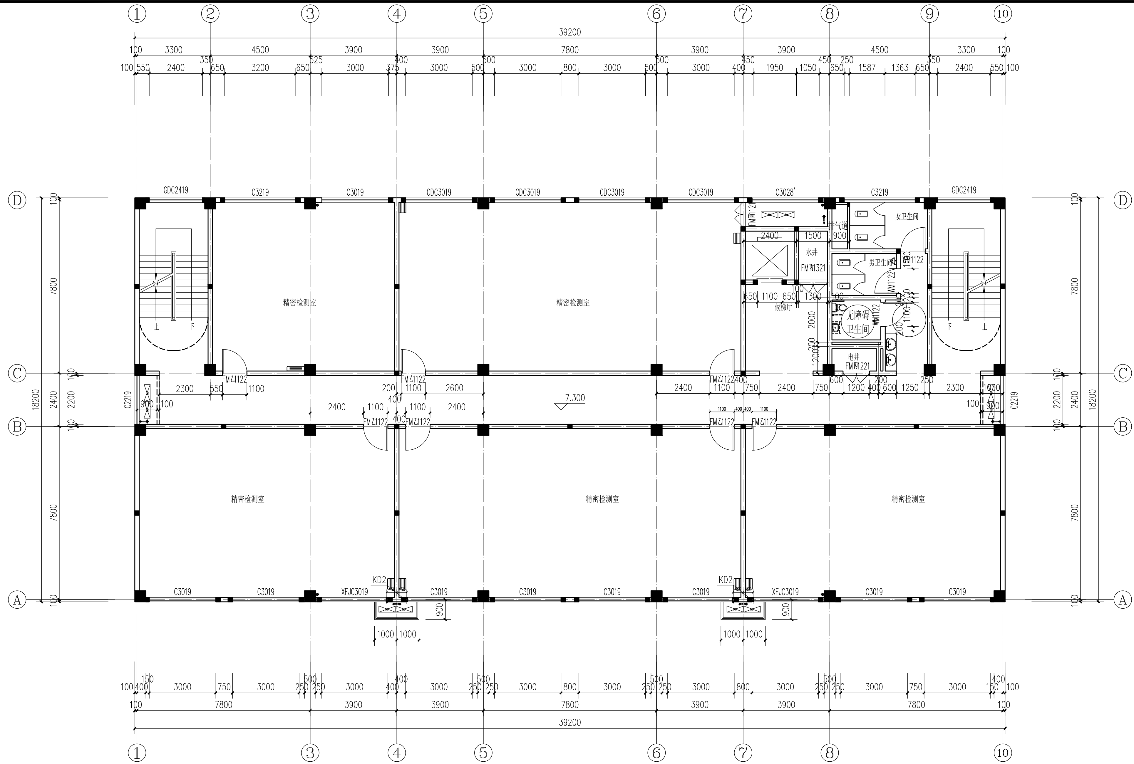
标准层平面图 1:100
