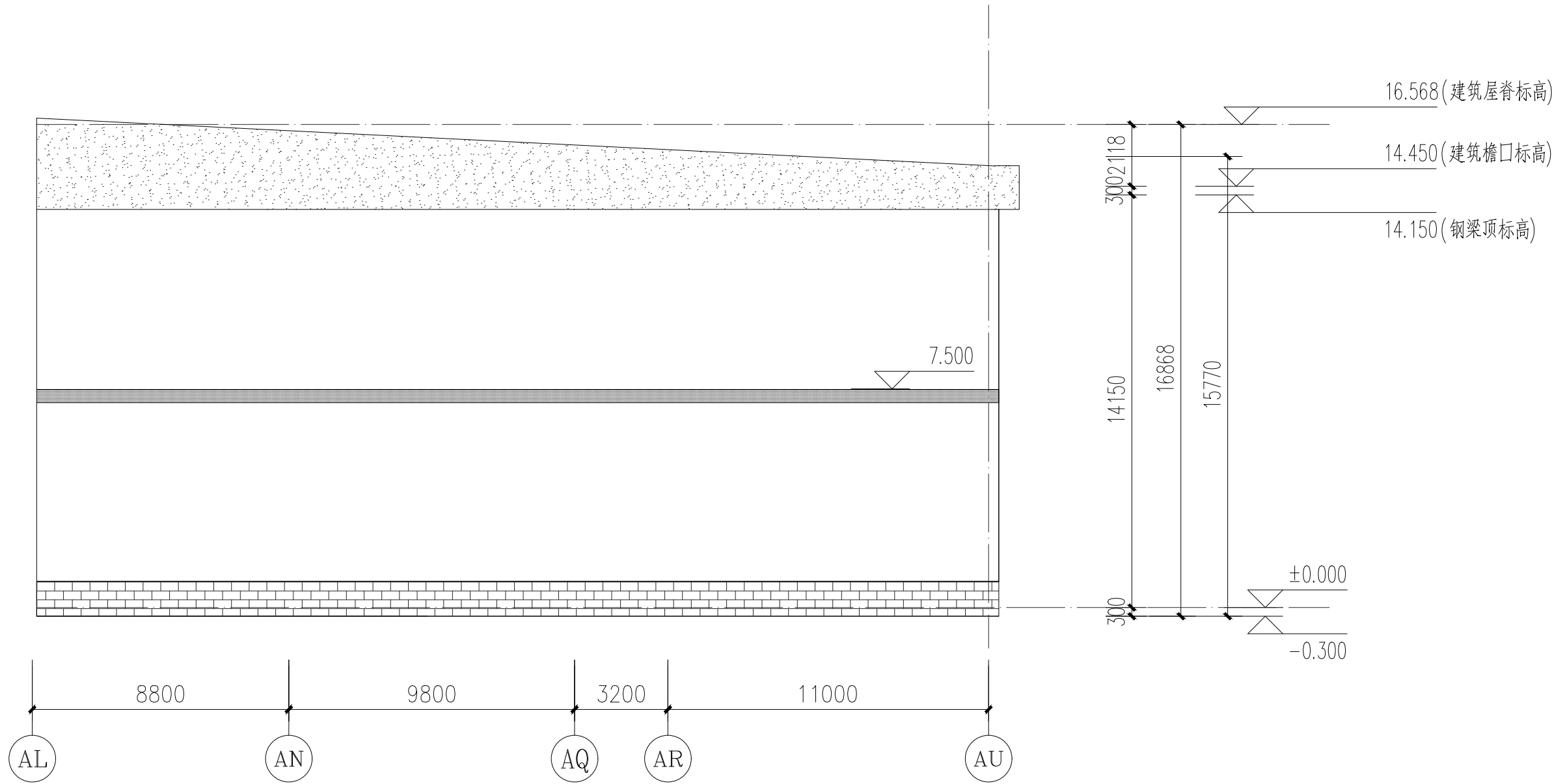
极片2 24 轴凹口位置立面图 1:250
