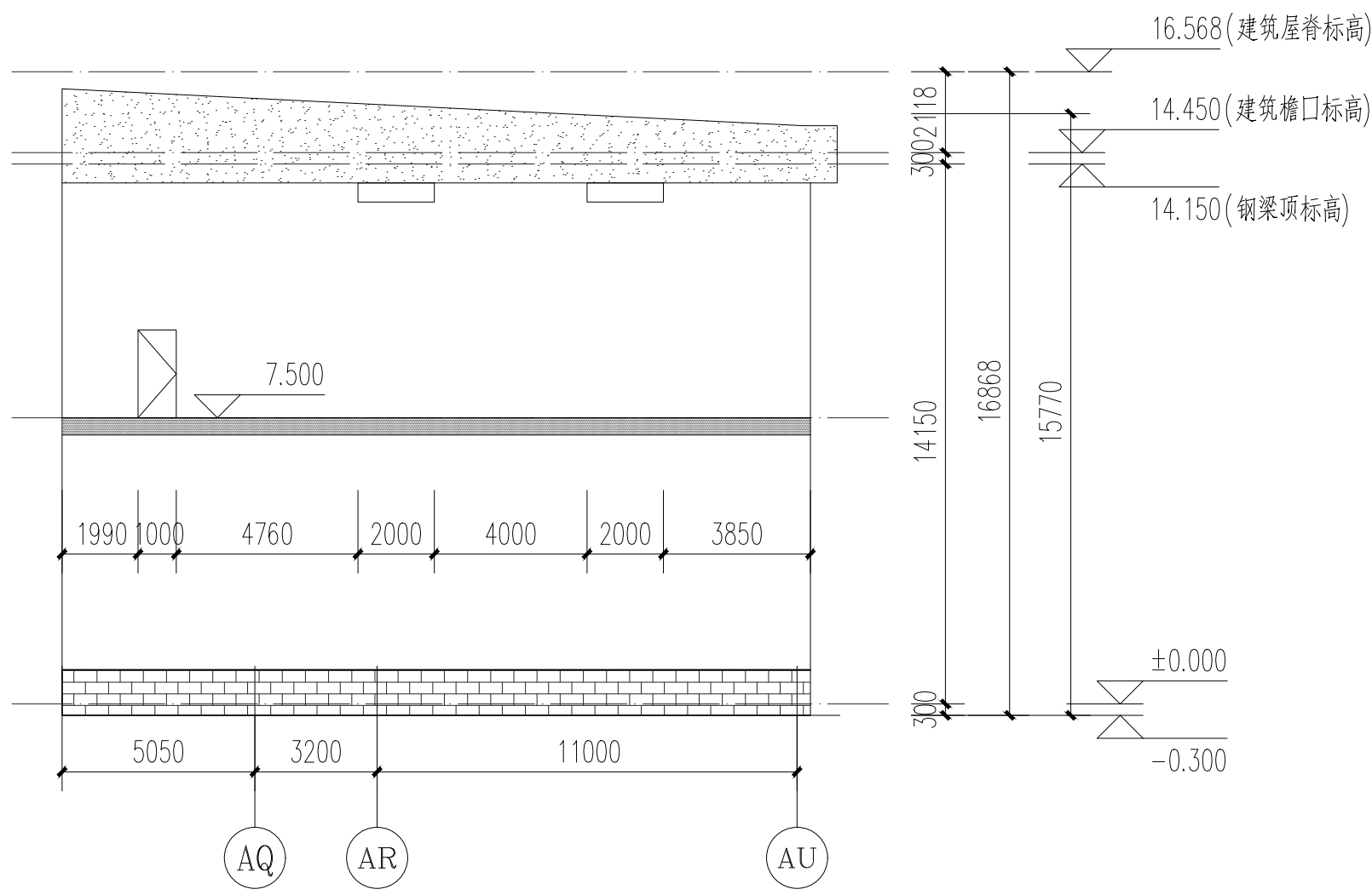
板片2 13轴凹口位置立面图 1:250
