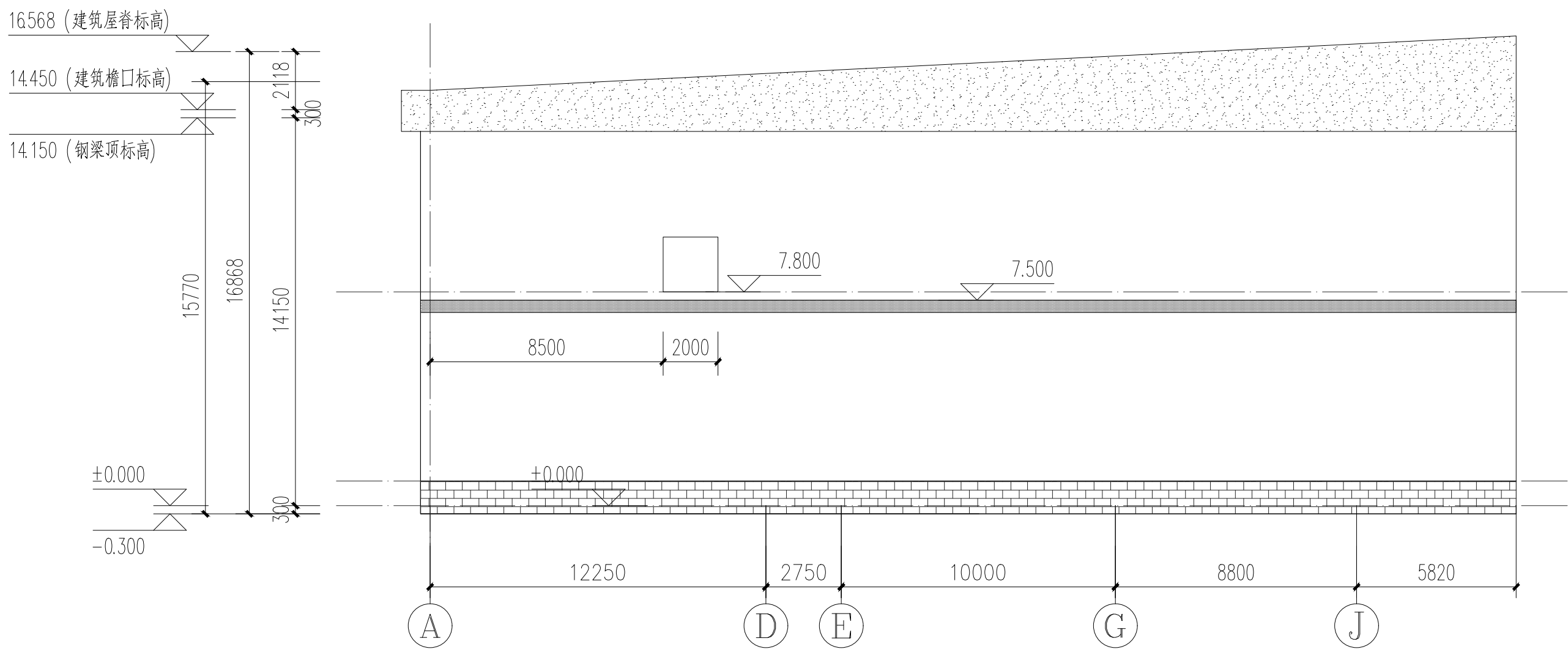
极片2 24 轴凹口位置立面图 1:250
