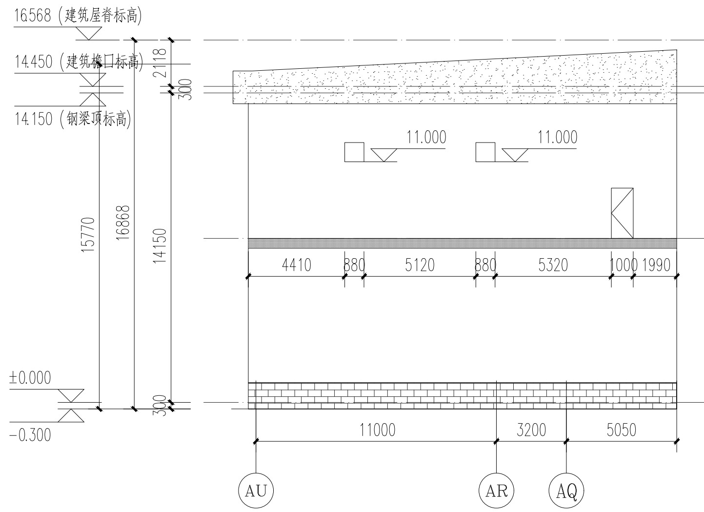
板片2 14轴凹口位置立面图 1:250
