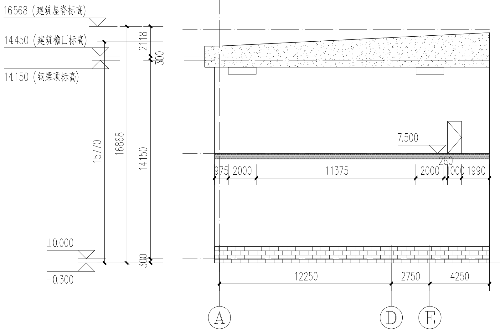
板片2 13 轴凹口位置立面图 1:250
