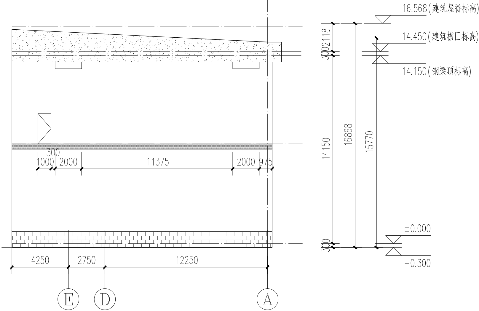
极片2 18 轴凹口位置立面图 1:250
