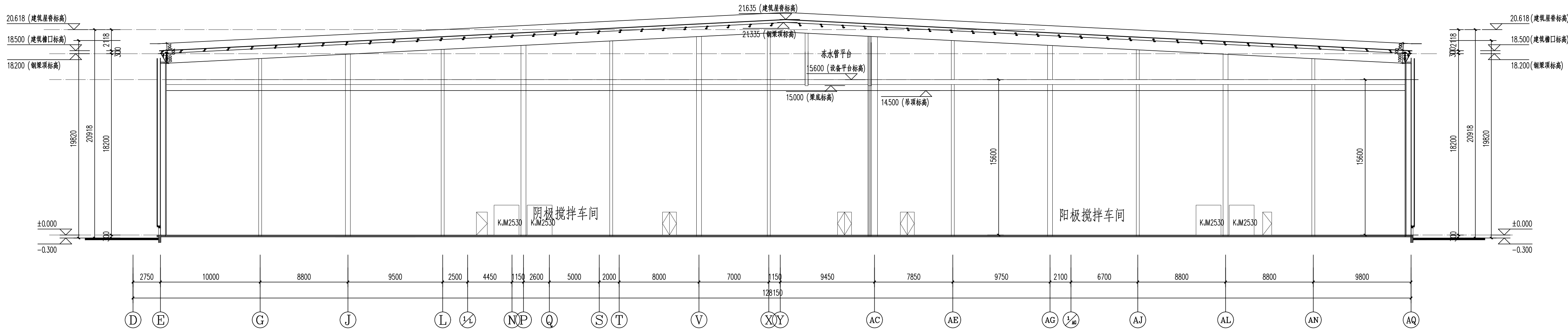
板片2 3-3剖面图(前工序搅拌车间) 1:200
