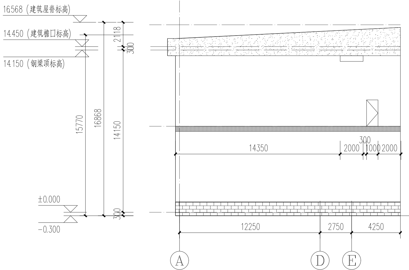
极片2 17 轴凹口位置立面图 1:250
