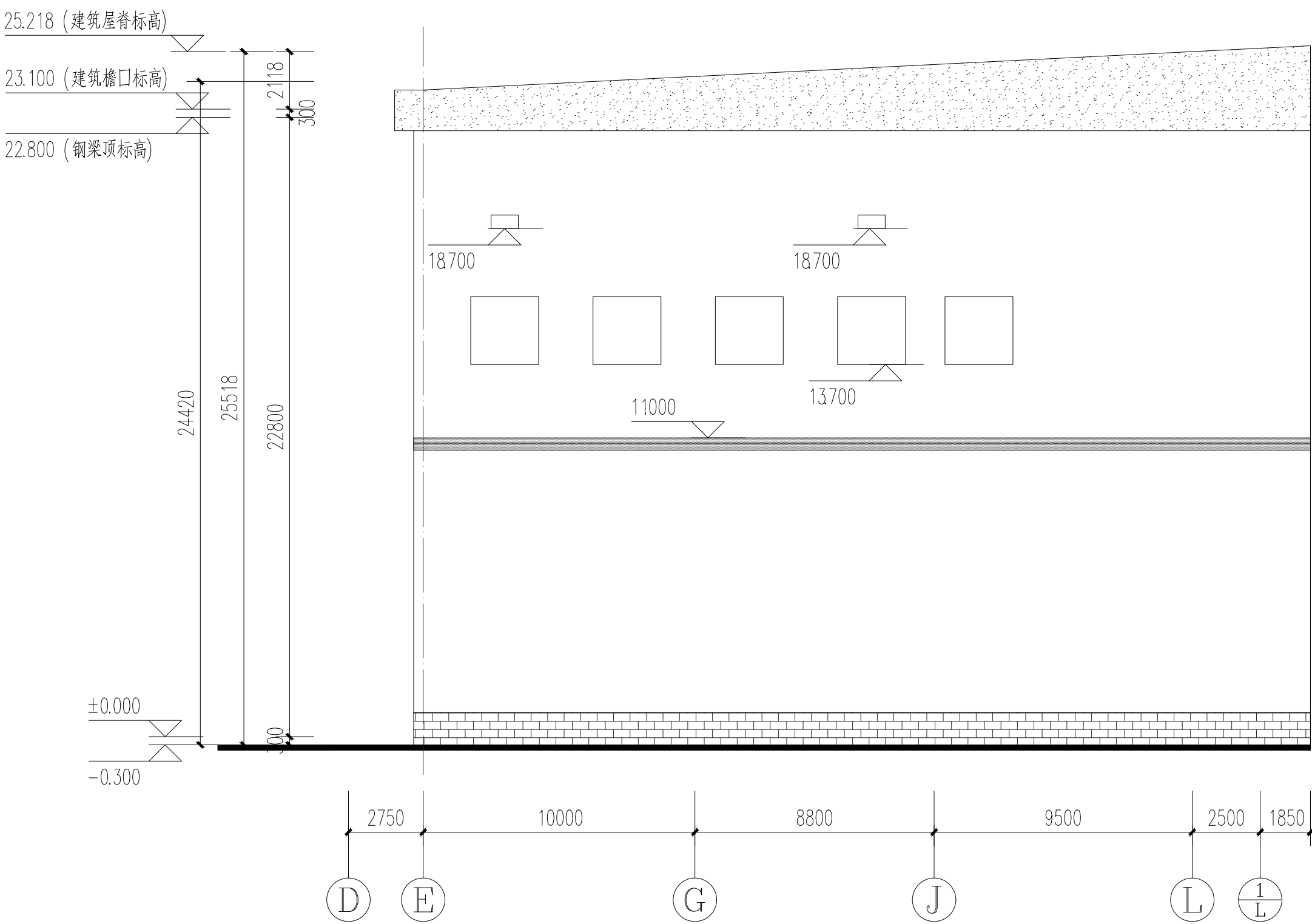
极片2 37 轴凹口位置立面图 1:250
