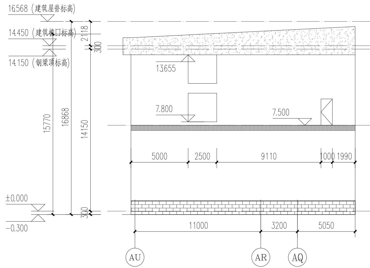
极片2 18 轴凹口位置立面图 1:250
