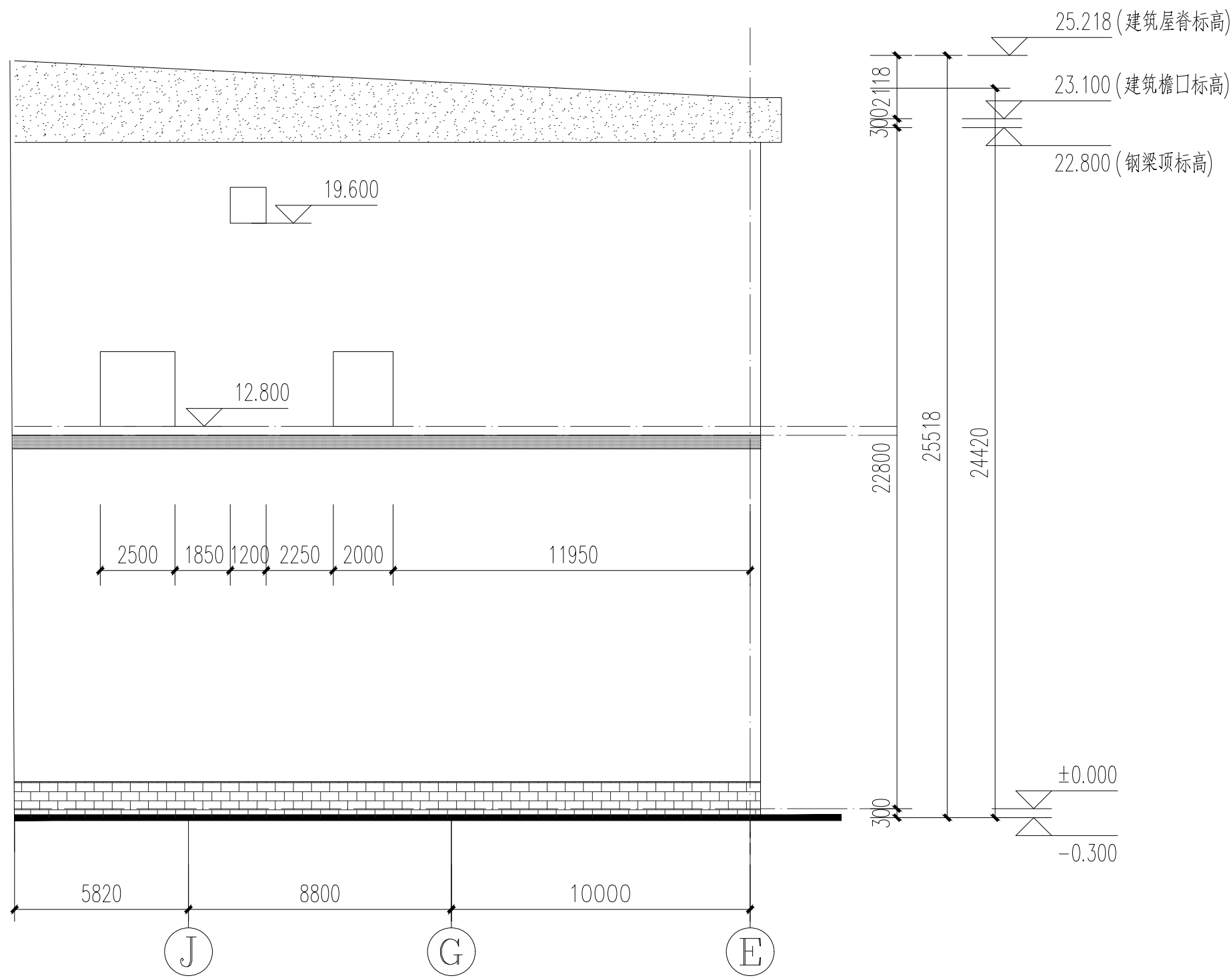
极片2 25 轴凹口位置立面图 1:250
