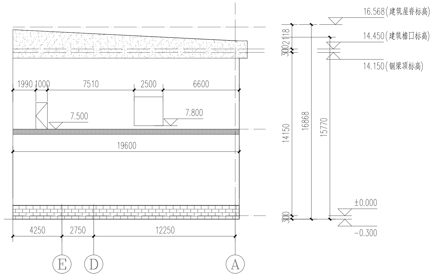
板片2 14轴凹口位置立面图 1:250
