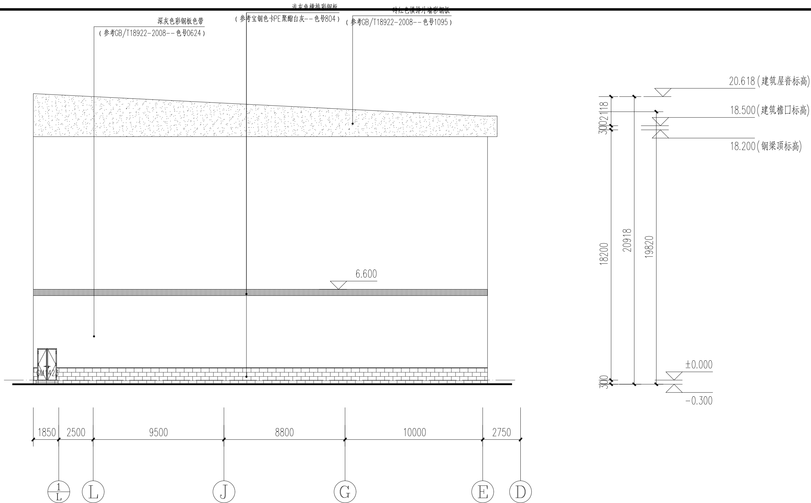
极片2 38轴凹口位置立面图 1:250
