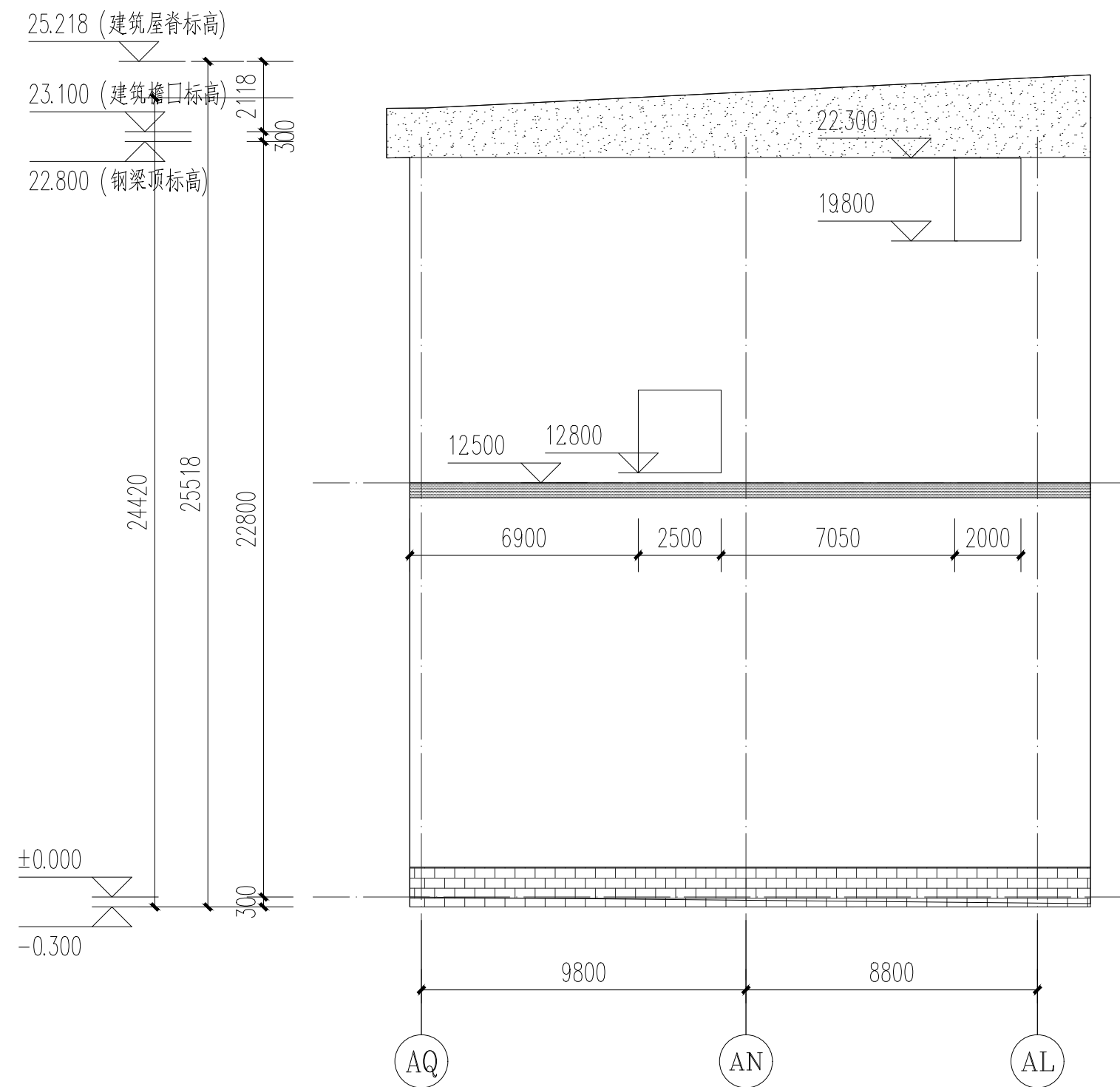
极片2 25 轴凹口位置立面图 1:250
