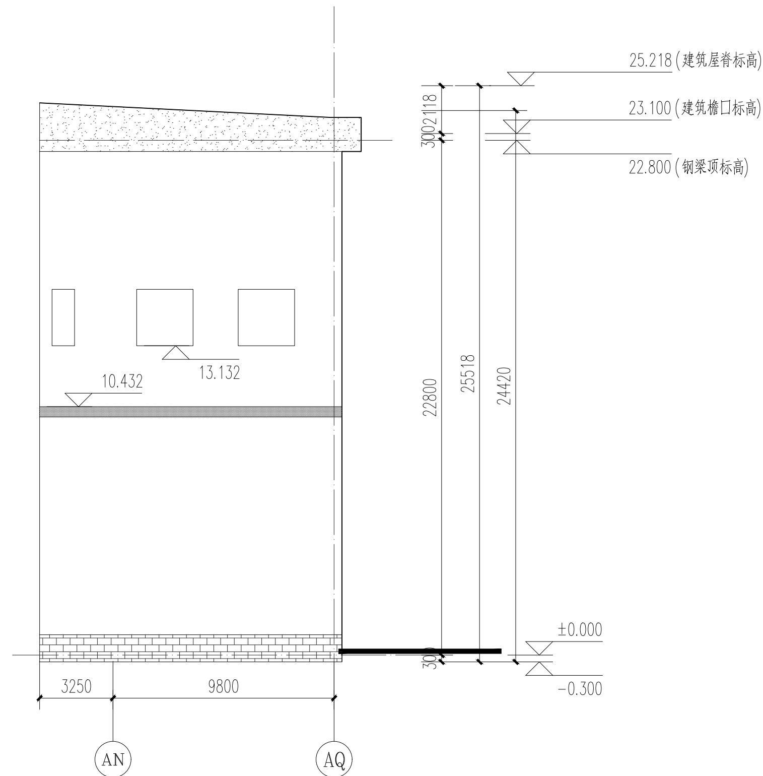
极片2 37轴凹口位置立面图 1:250
