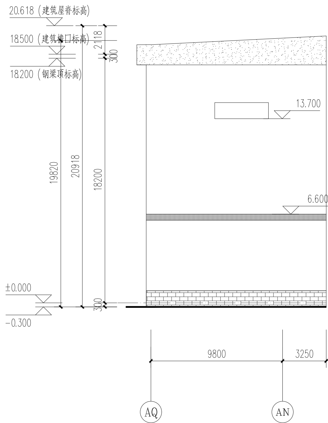
极片2 38轴凹口位置立面图 1:250
