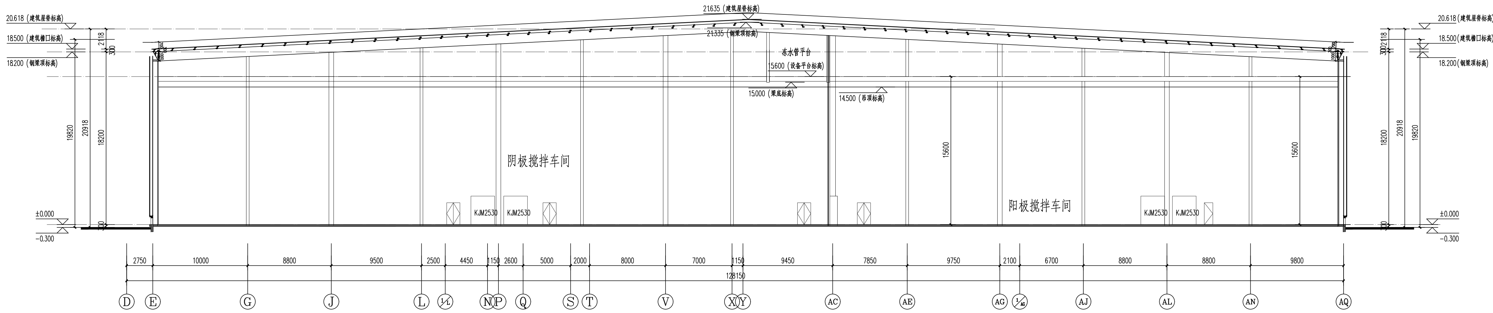
板片2 4-4剖面图(凹版车间) 1:200
