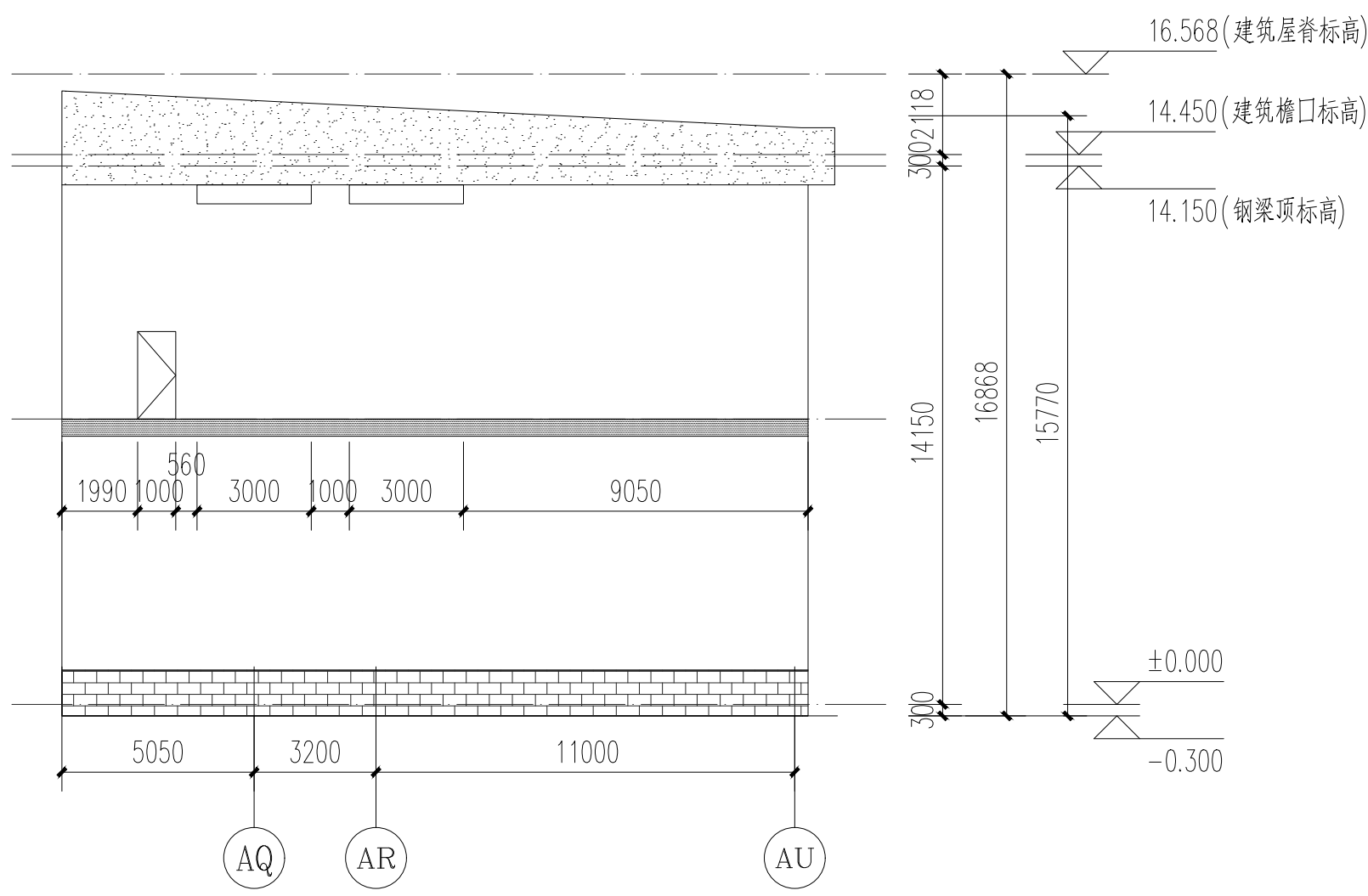
极片2 17 轴凹口位置立面图 1:250
