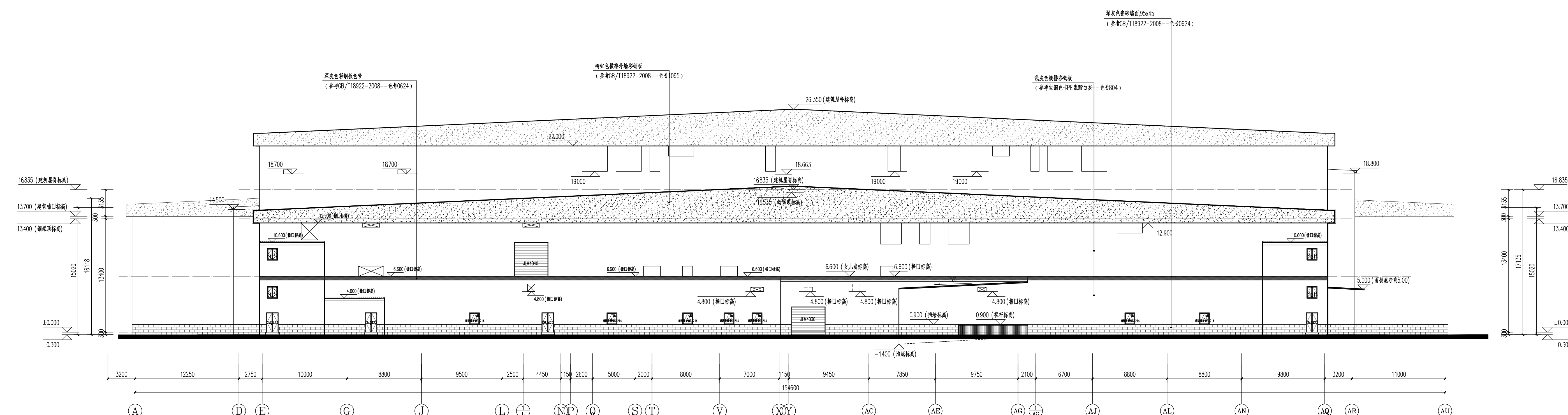
①-⑭轴立面图 1:250
