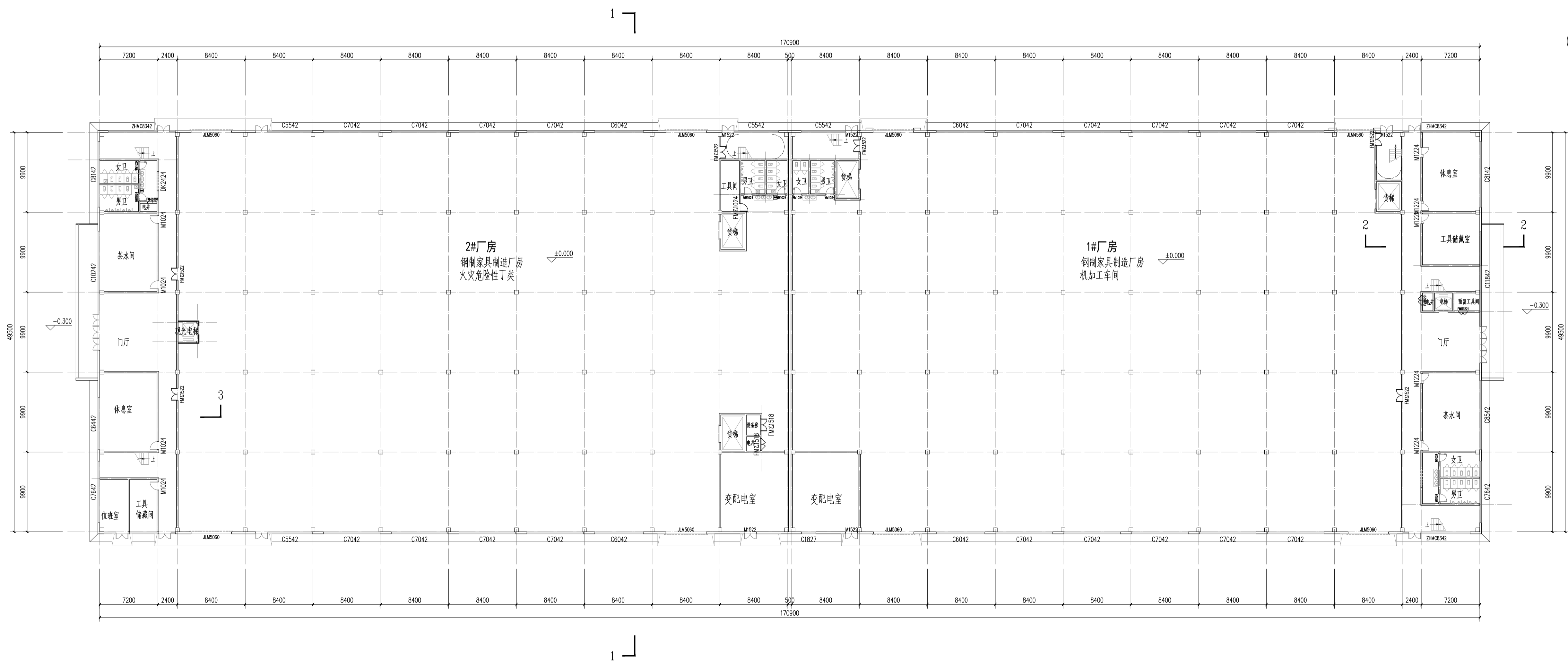
2#厂房一层平面图 1:200
