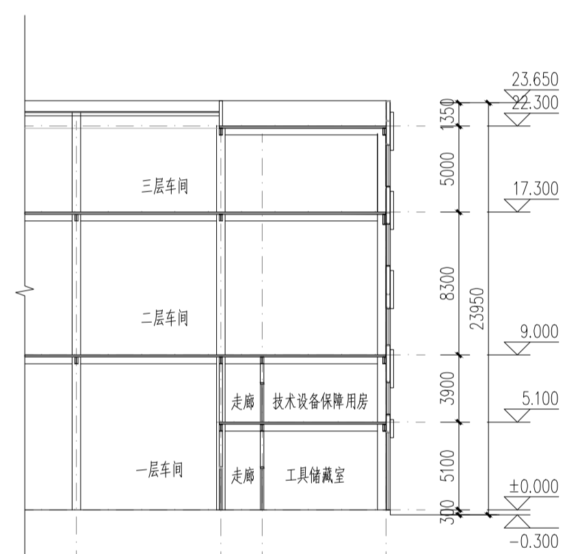
2-2剖面图 1:200
