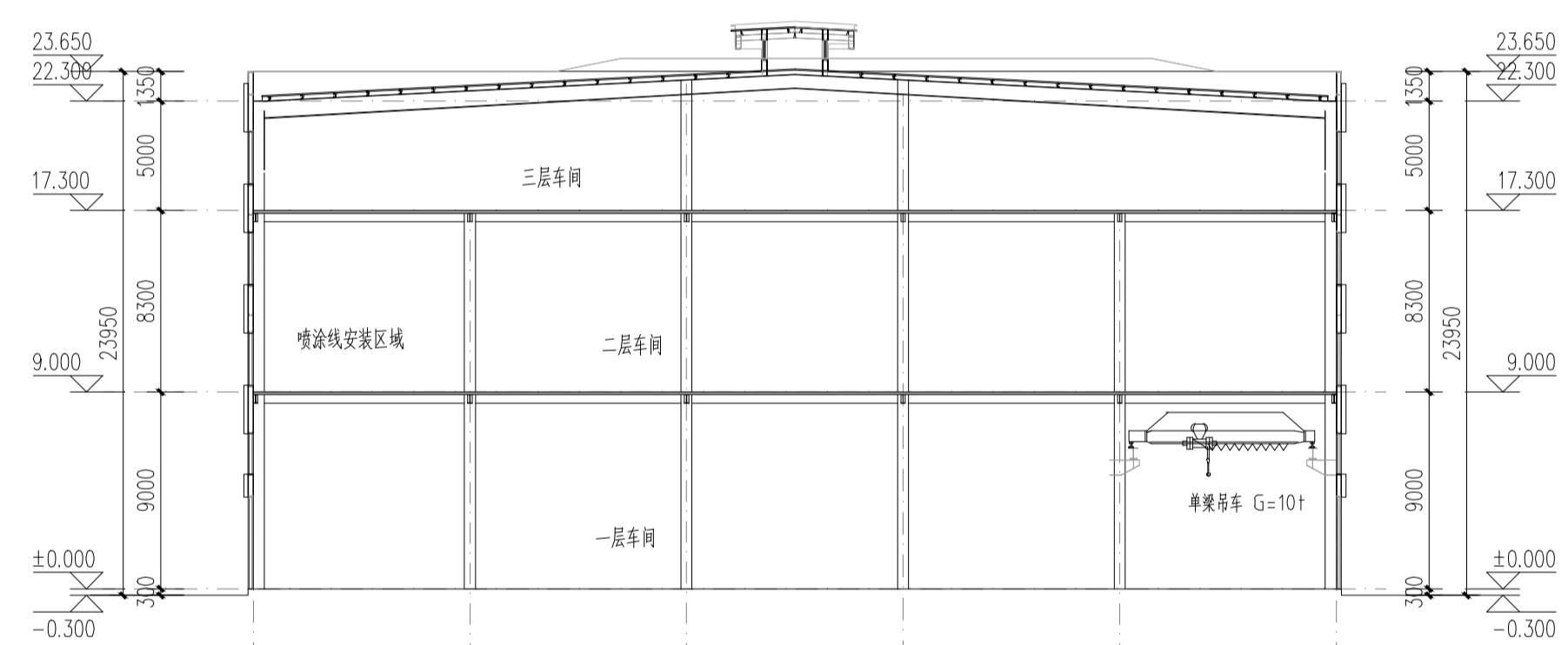
1-1剖面图 1:200
