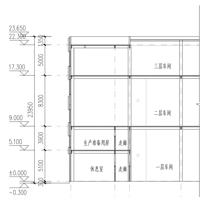
3-3剖面图 1:200
