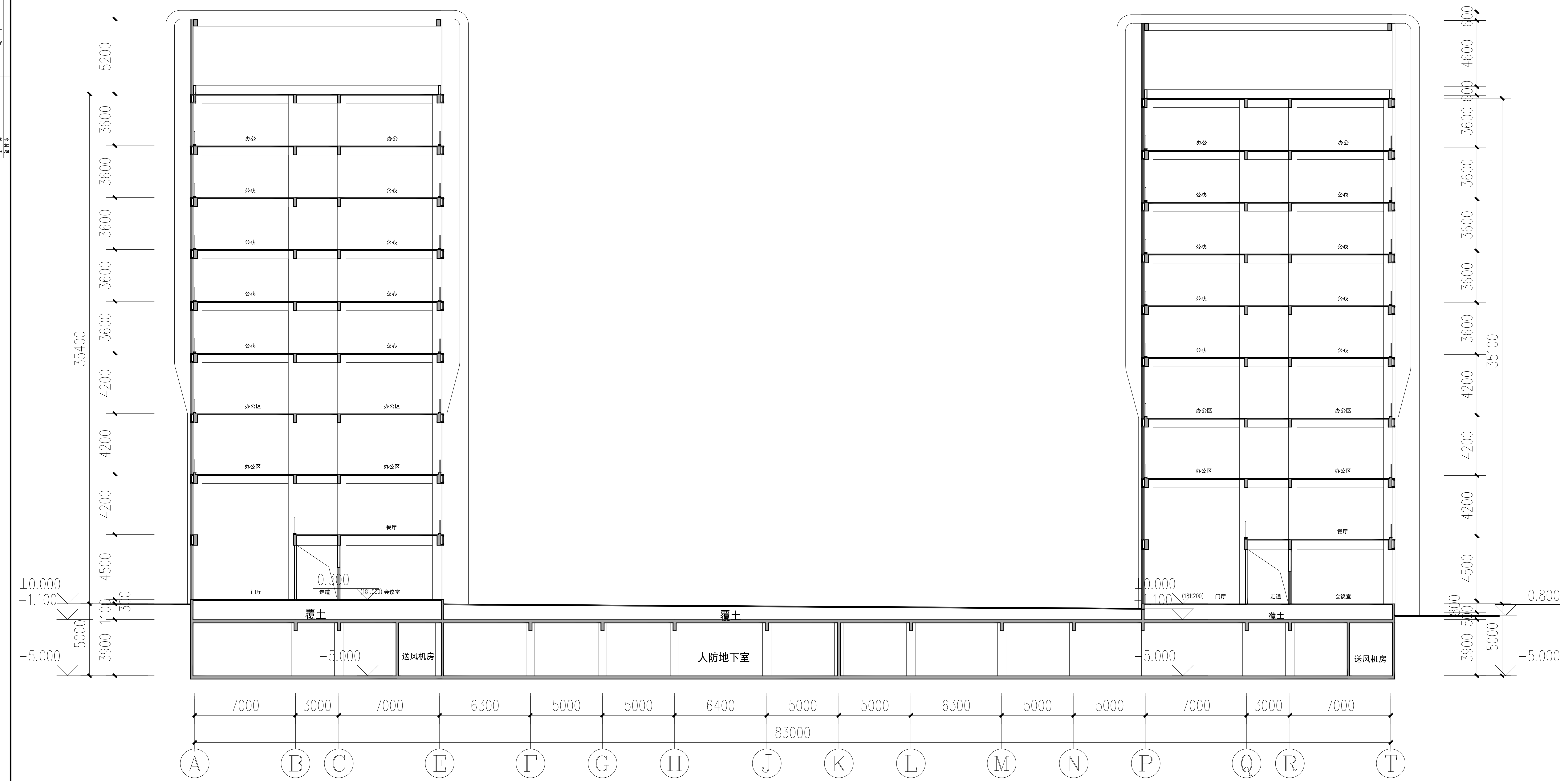
2-2剖面图
