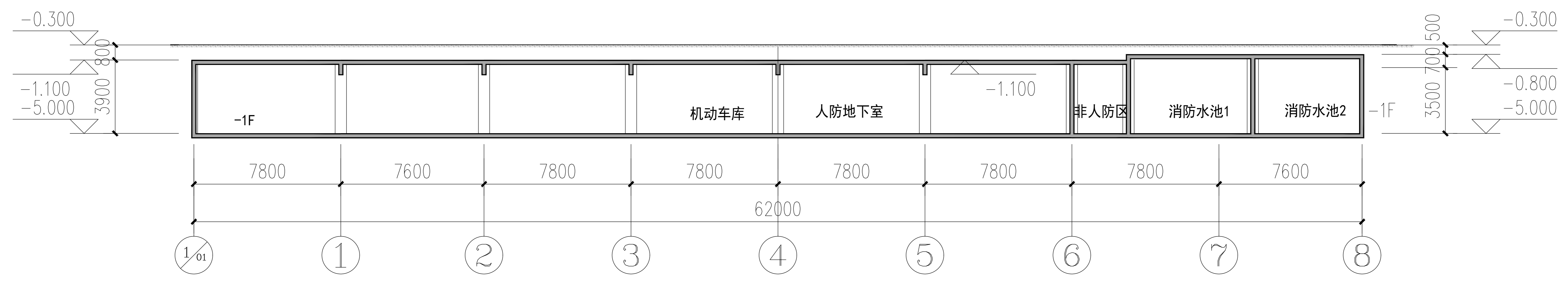
1-1剖面图
