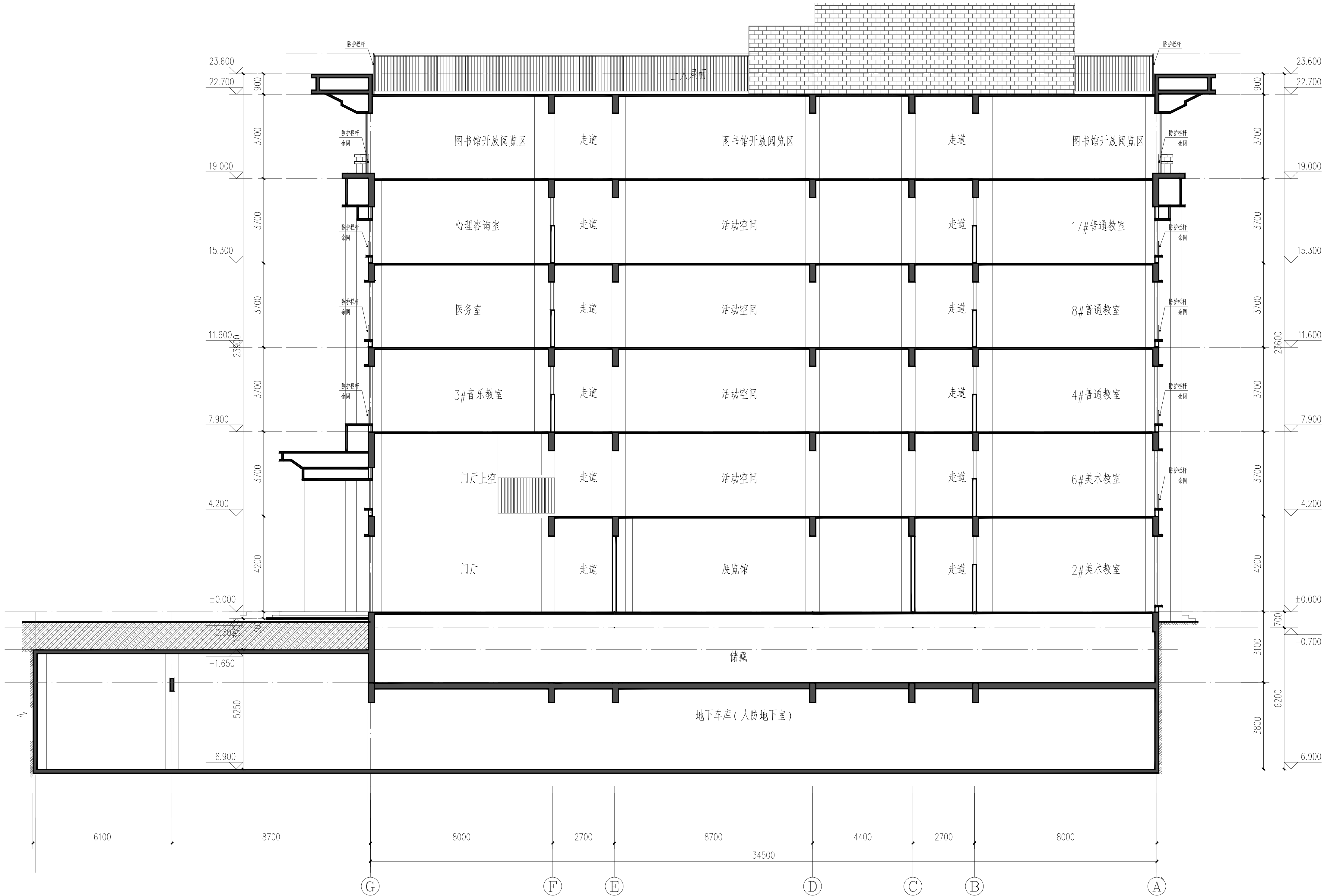
1-1 剖面图 1:100
