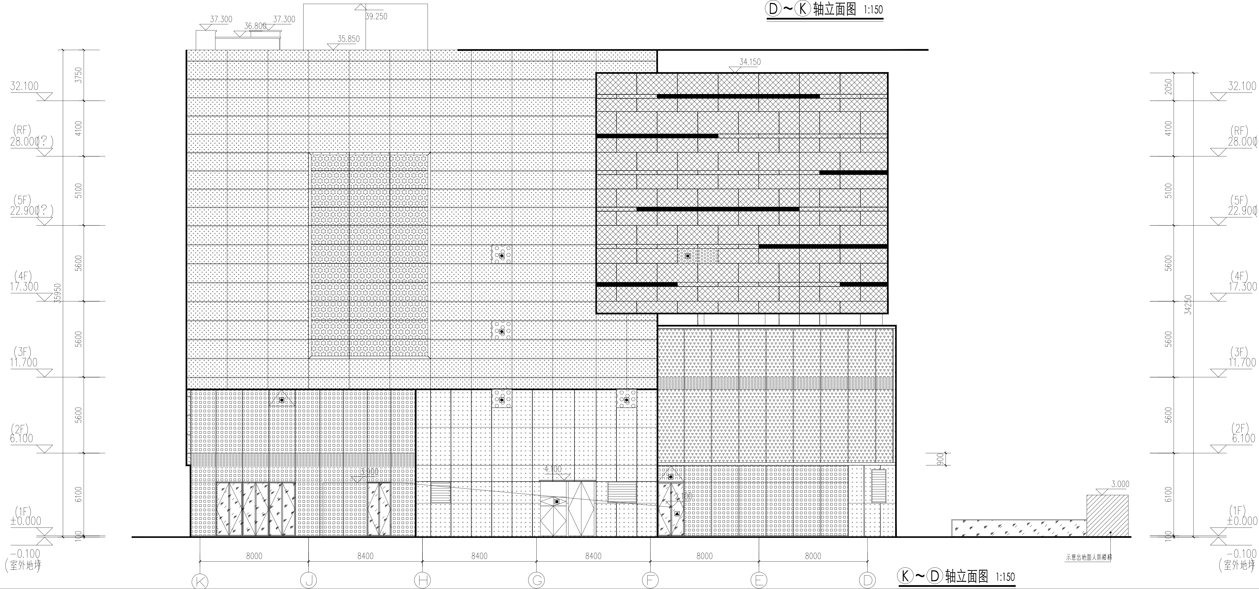
D~K 轴立面图 1:150
