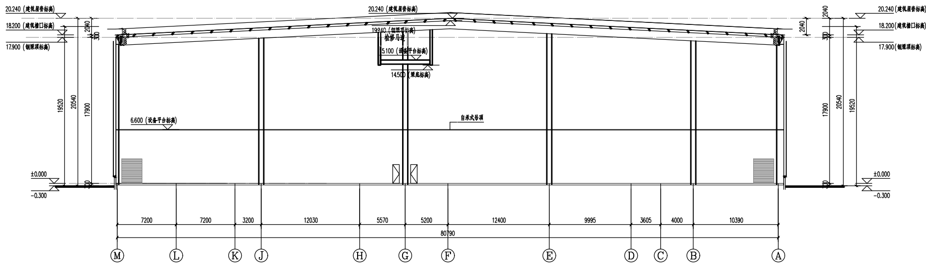
板片1 2-2剖面图 (粉料段) 1:200
