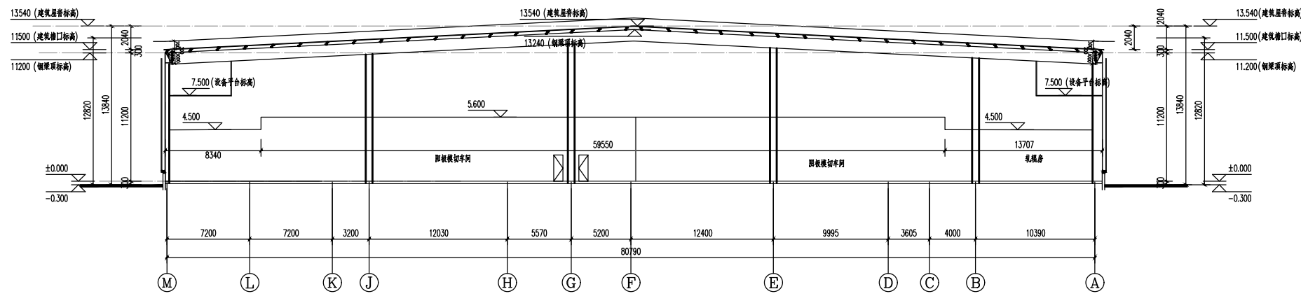
板片1 7-7 剖面图 (冷压车间) 1:200
