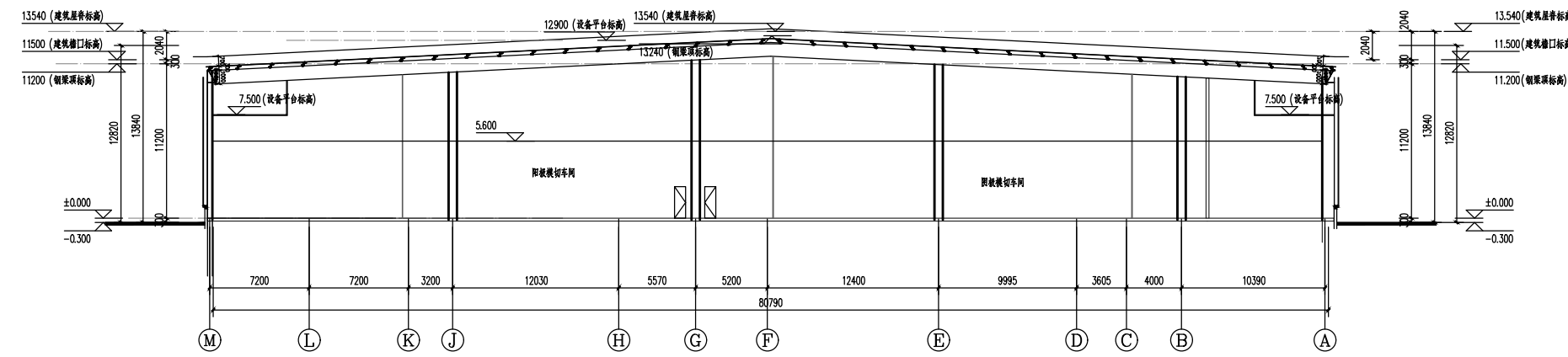
板片1 8-8 剖面图 (板片模切车间) 1:200
