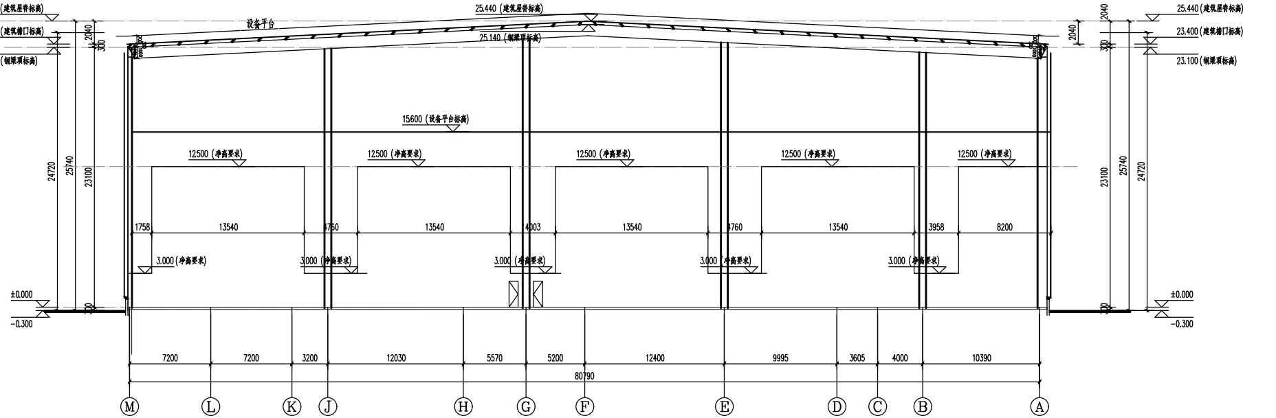
板片1 5-5剖面图 (涂布烘箱段) 1:200
