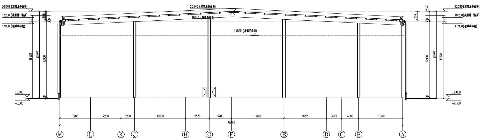
板片1 3-3剖面图 (搅拌段) 1:200
