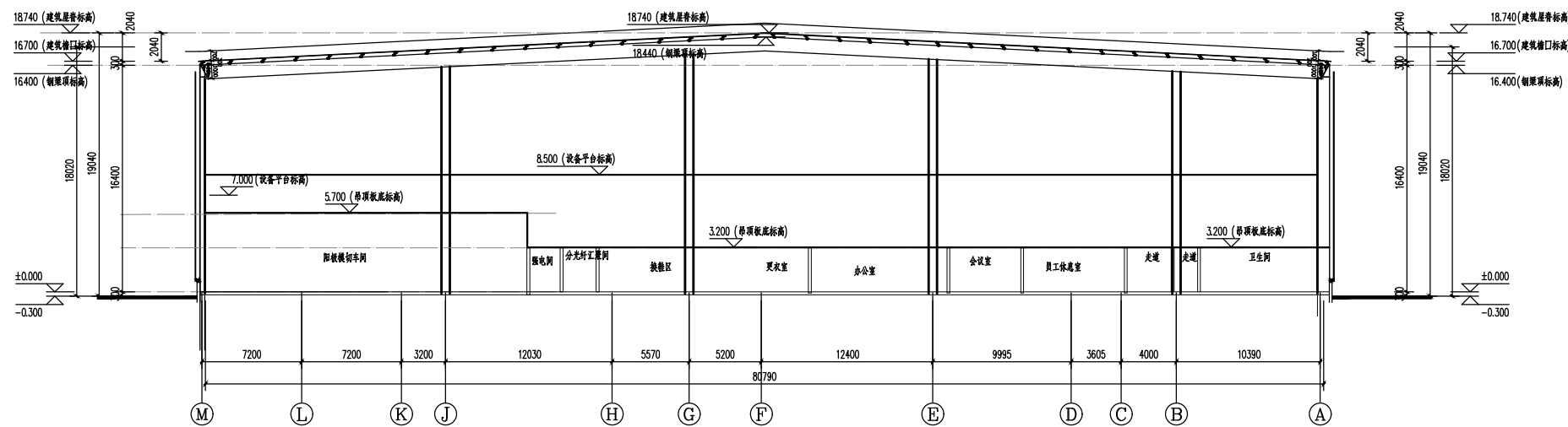
板片1 9-9 剖面图 (辅房) 1:200
