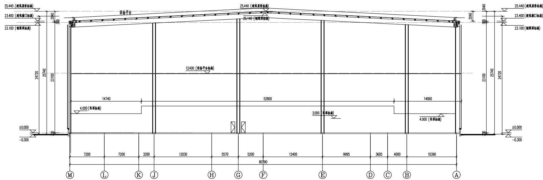
板片1 6-6 剖面图 (板片冷压车间) 1:200
