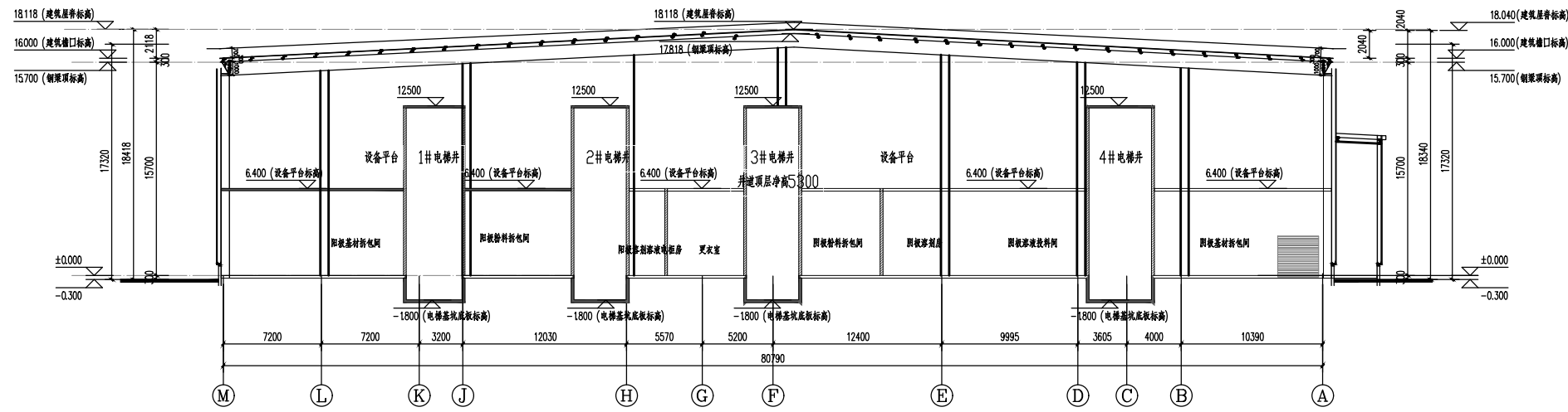
板片1 1-1剖面图 (前工序辅房段) 1:200
