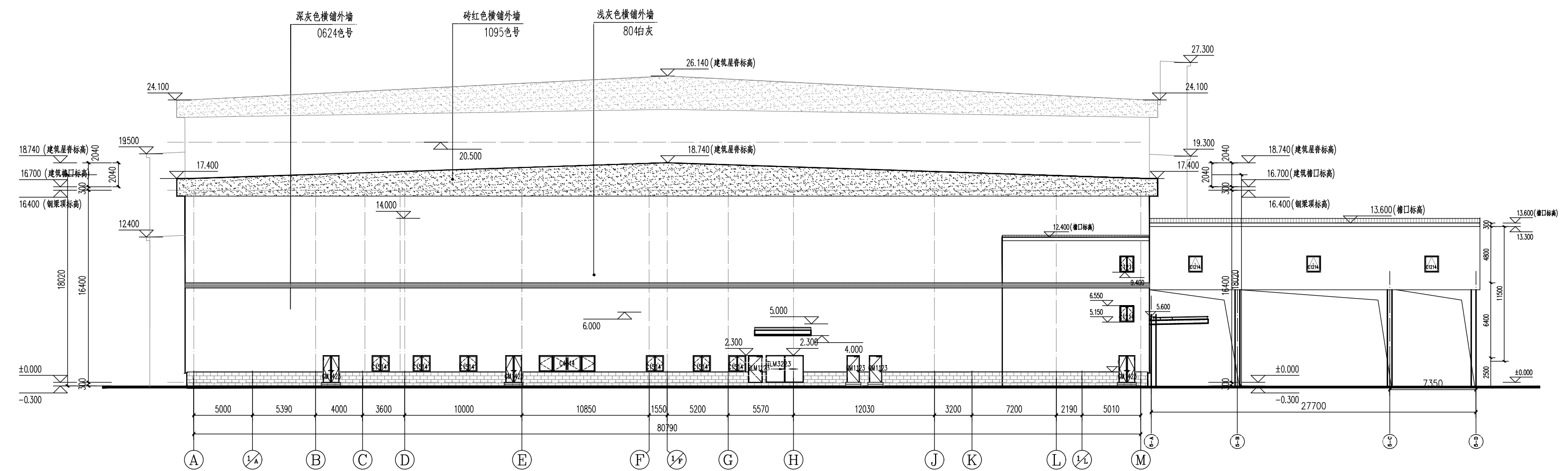
板片1 A轴~M轴立面图
