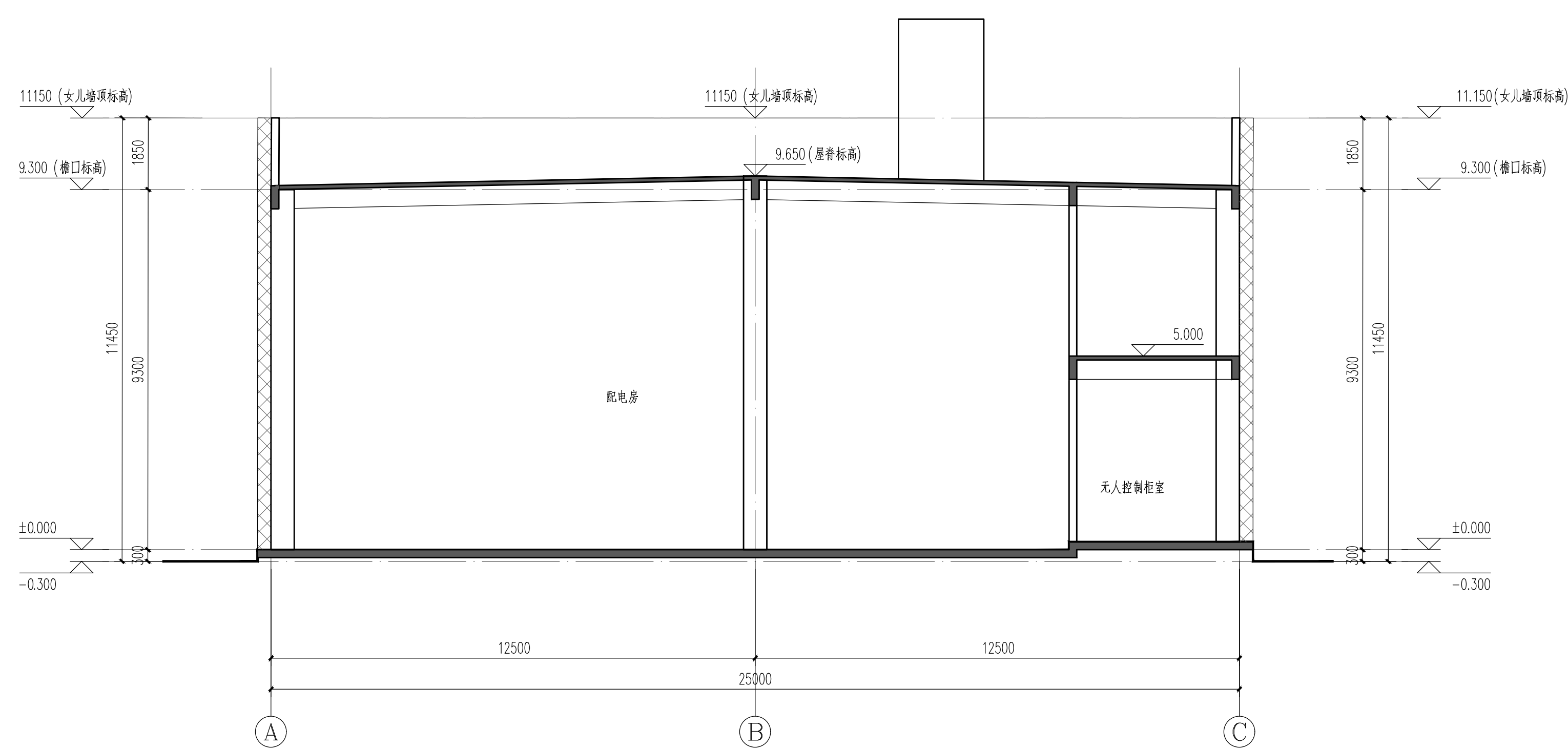
设施房3 2-2剖面图 1:100
