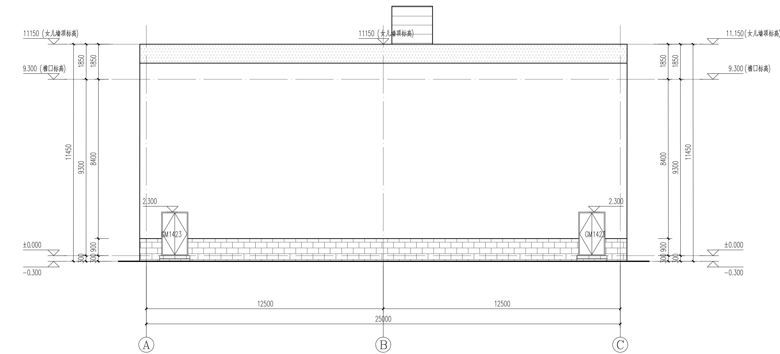
设施房3 (A)-③轴立面图 1:100
