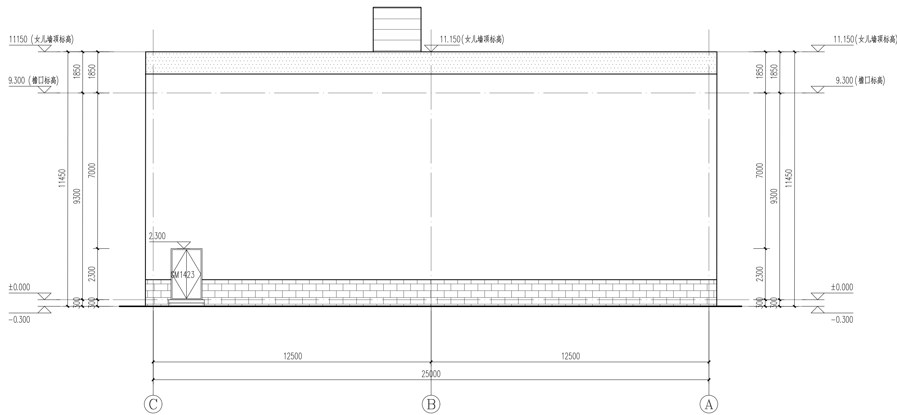
设施房3 ③-(A)轴立面图 1:100
